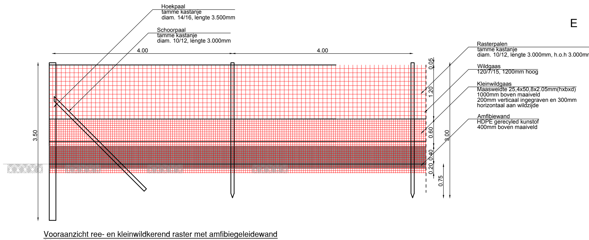
Voorwaanzicht ree- en kleinwiderend raster met afbieg geleidewand Schaal 1:50
