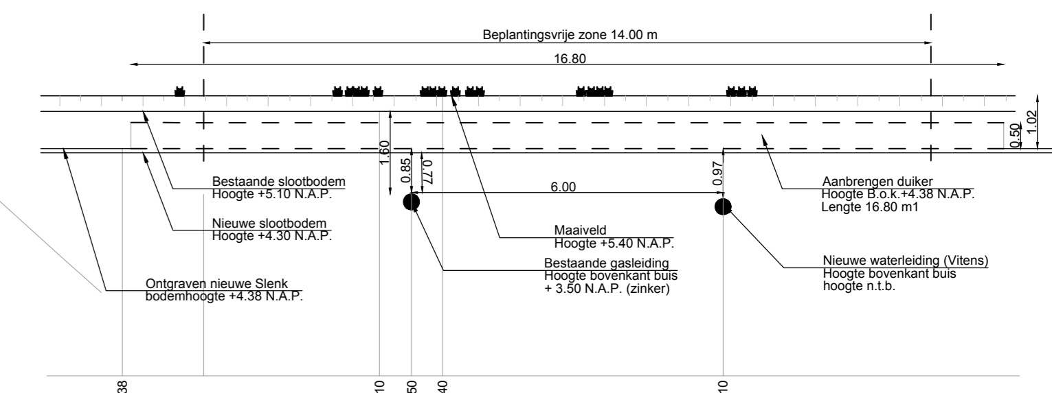
Kruising Gaesdijk en Waterleiding Viars met Slenk Schaal 1:100
