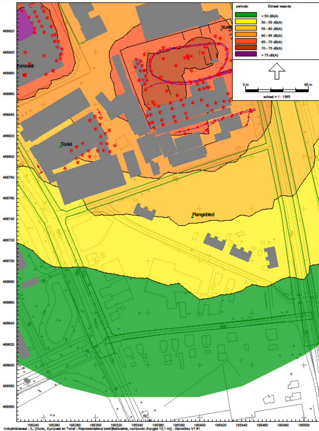
Representatieve bedrijfssituatie Vurec, Eurocast en Toriel (vergund) cumulatieve etmaalwaarde countouren (hoogte 13,1 m boven het maaiveld)
