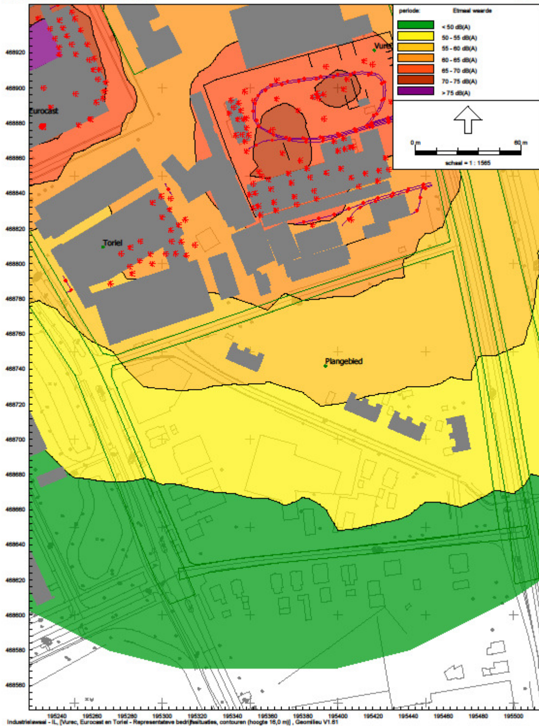
Representatieve bedrijfssituatie Vurec, Eurocast en Toriel (vergund) cumulatieve etmaleelwaarde countouren (hoogte 16.0 m boven het maaiveld)
