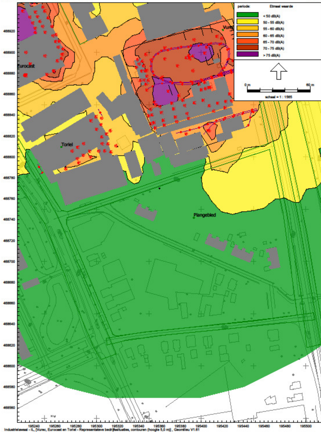
Representatieve bedrijfssituatie Vurec, Eurocast en Toriel (vergund) cumulatieve etmaalwaardecontouren (hoogte 5,0 m boven het maaiveld)
