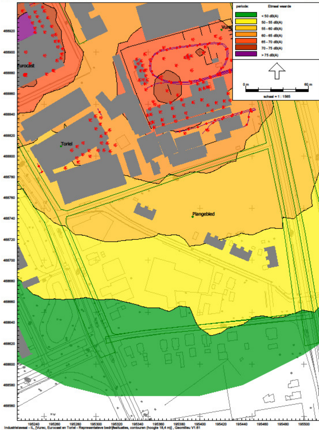
Representatieve bedrijfssituatie Vurec, Eurocast en Toriel (vergund) cumulatieve etmaalwaarde countouren (hoogte 18.4 m boven het maaiveld)
