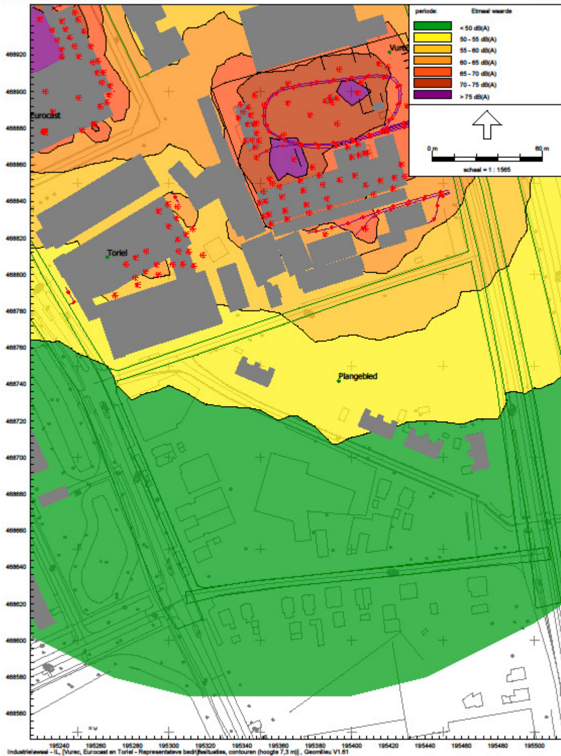
Representatieve bedrijfssituatie Vurec, Eurocast en Toriel (vergund) cumulatieve etmaalwaarde countouren (hoogte 7.3 m boven het maaiveld)
