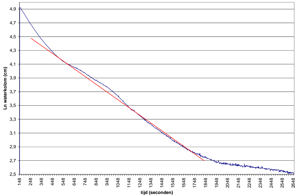
Infiltratiegrafiek De Heurne Ln (waterkolom) boring 04, proef 1
