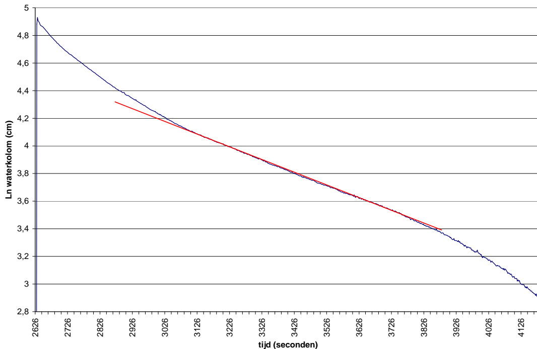
Infiltratiegrafiek De Heurne Ln (waterkolom) boring 01, proef 1
