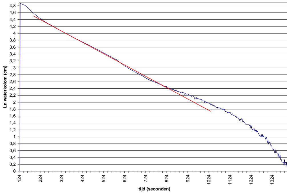
Infiltratiegrafiek De Heurne Ln (waterkolom) boring 06, proef 1
