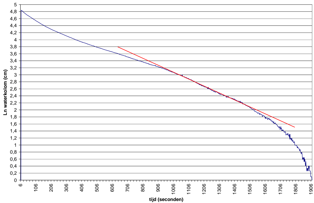
Infiltratiegrafiek De Heurne Ln (waterkolom) boring 05, proef 1
