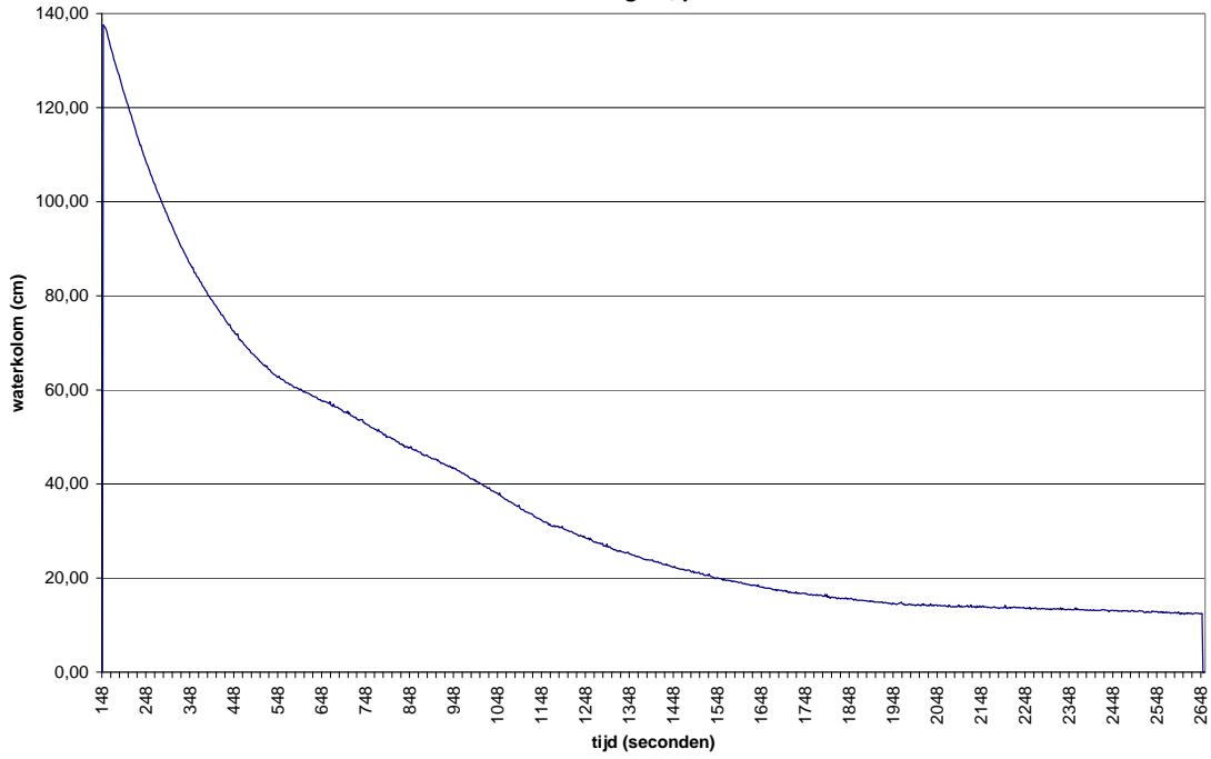
Aalten, De Heurne boring 04, proef 1
