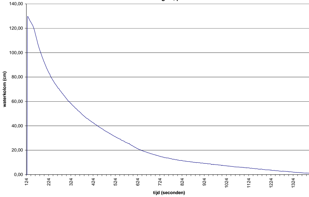
Aalten, De Heurne boring 06, proef 1
