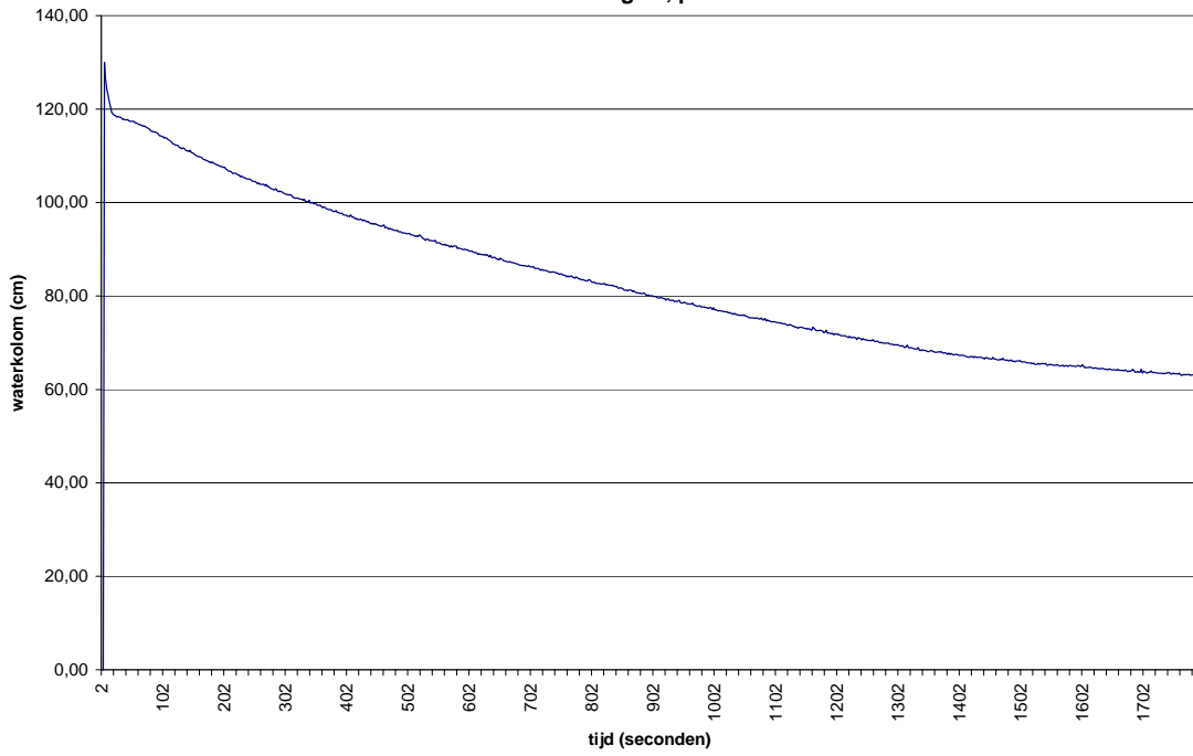
Aalten, De Heurne boring 02, proef 2
