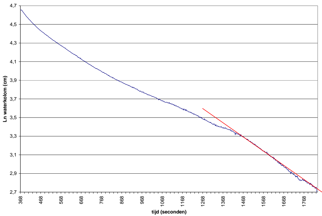
Infiltratiegrafiek De Heurne Ln (waterkolom) boring 03, proef 1
