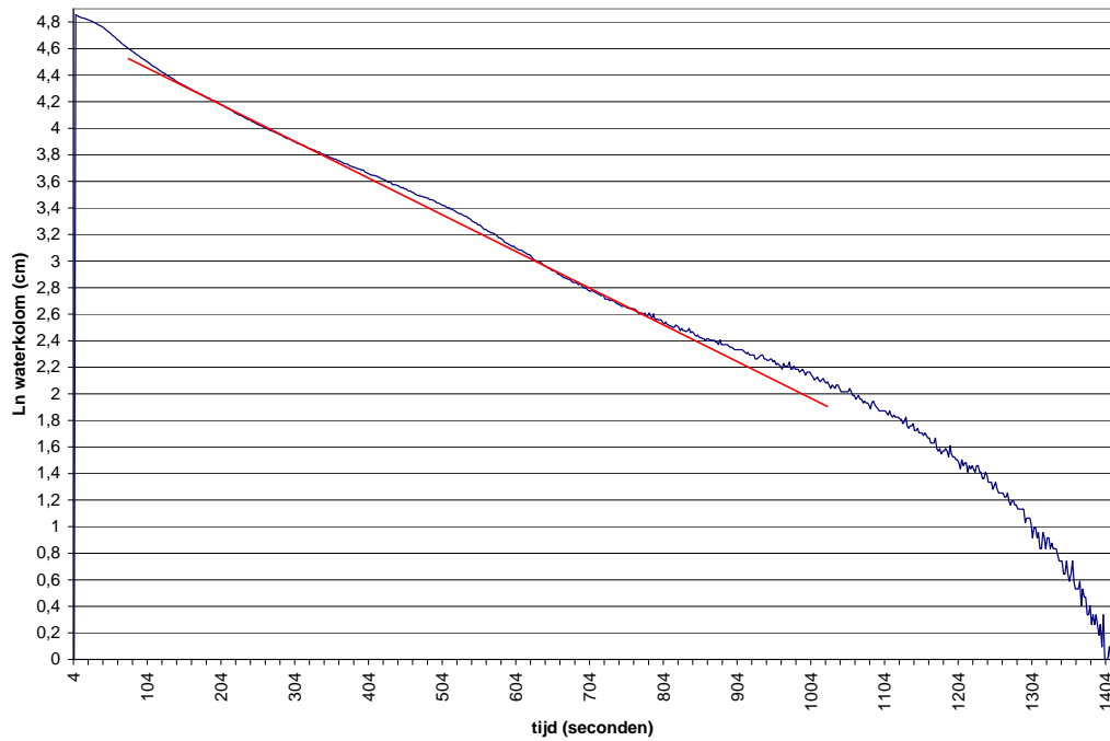
Infiltratiegrafiek De Heurne Ln (waterkolom) boring 06, proef 2
