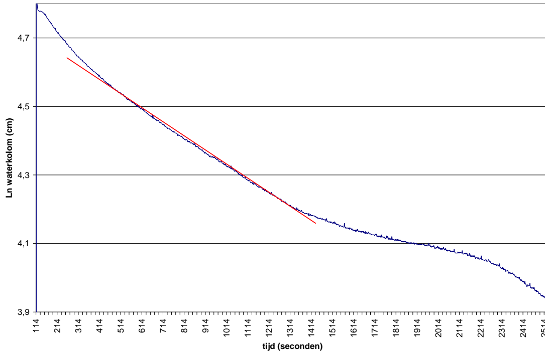
Infiltratiegrafiek De Heurne Ln (waterkolom) boring 02, proef 1
