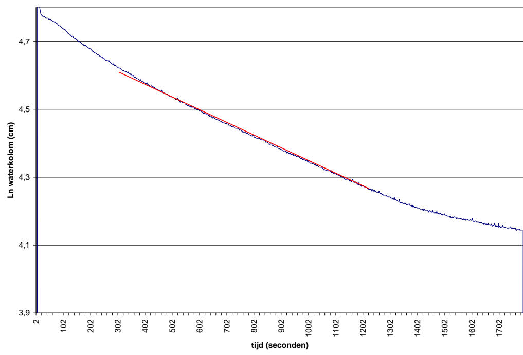
Infiltratiegrafiek De Heurne Ln (waterkolom) boring 02, proef 2
