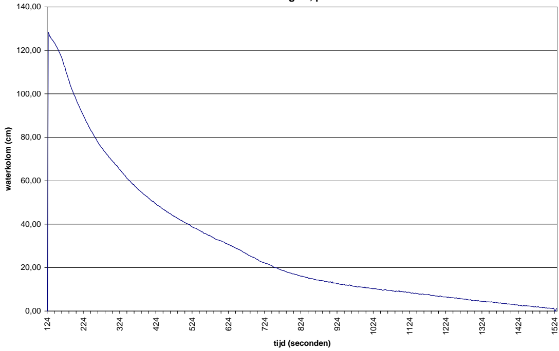
Aalten, De Heurne boring 06, proef 2
