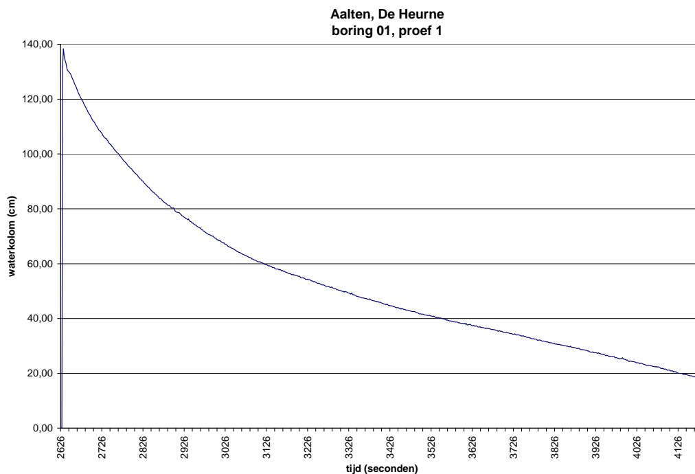
Figuur 2 Infiltratiecurve proef 1
