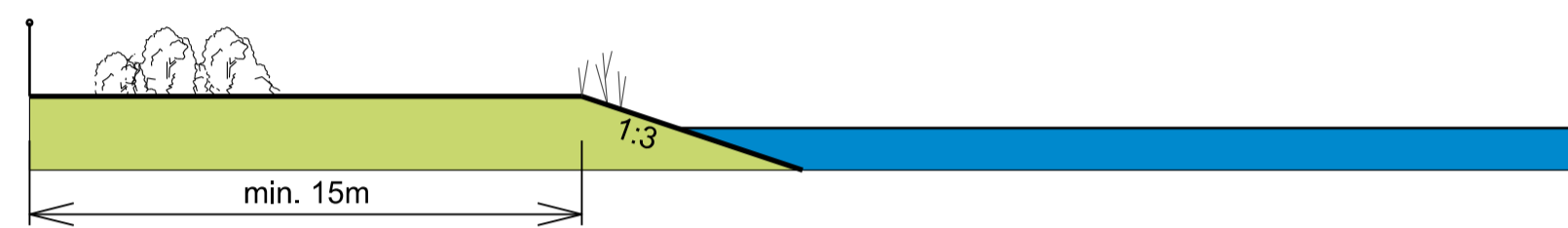
Dwarsprofiel 3 schaal 1:200
