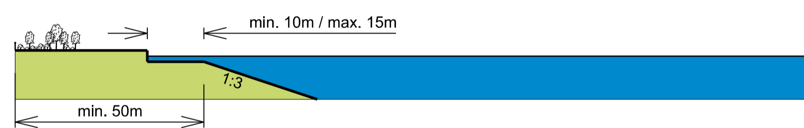
Dwarsprofiel 6 schaal 1:1000
