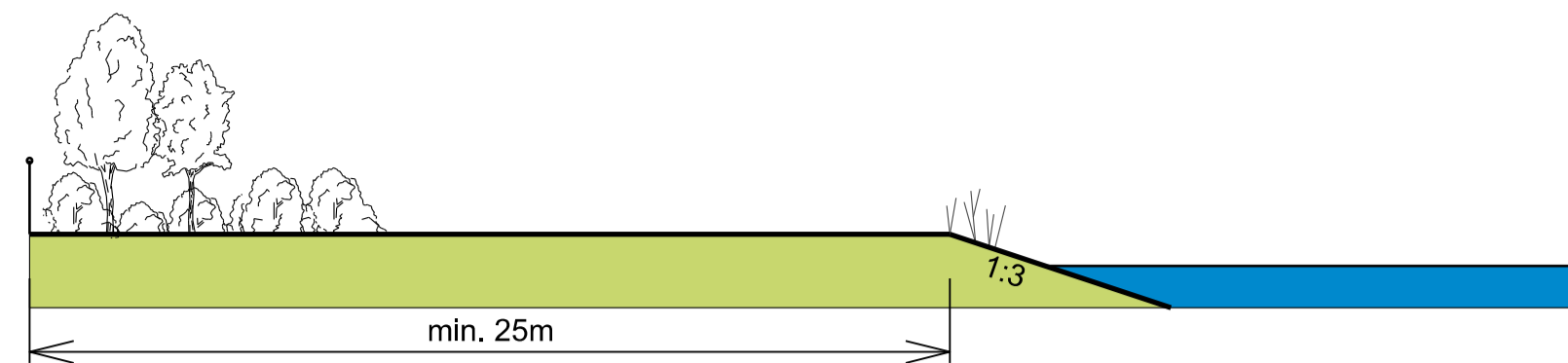
Dwarsprofiel 1 schaal 1:200
