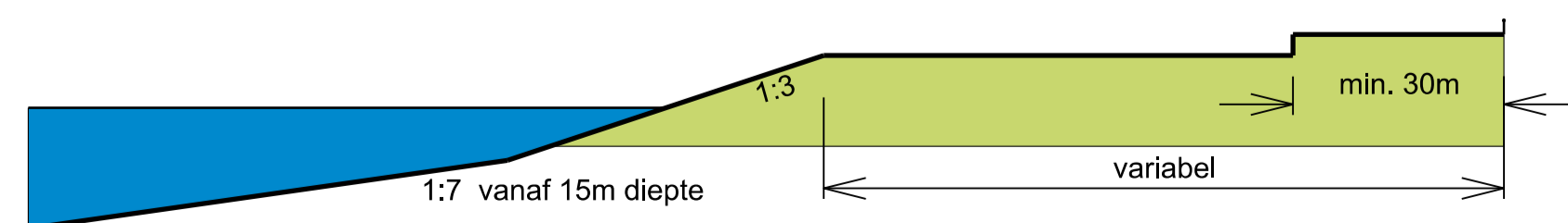
Dwarsprofiel 8 schaal 1:1000
