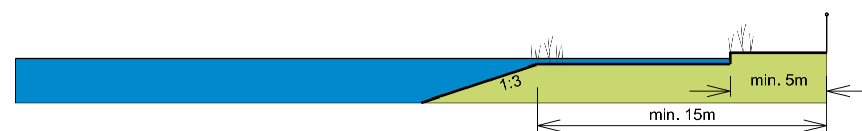
Dwarsprofiel 4 schaal 1:200
