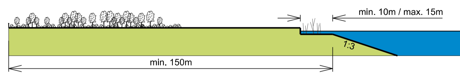
Dwarsprofiel 5 schaal 1:1000
