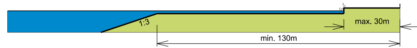
Dwarsprofiel 2 schaal 1:1000
