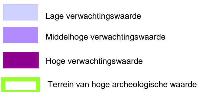
Uitsnede gemeentelijke archeologische verwachtings- en beleidsadvieskaart Heeten
