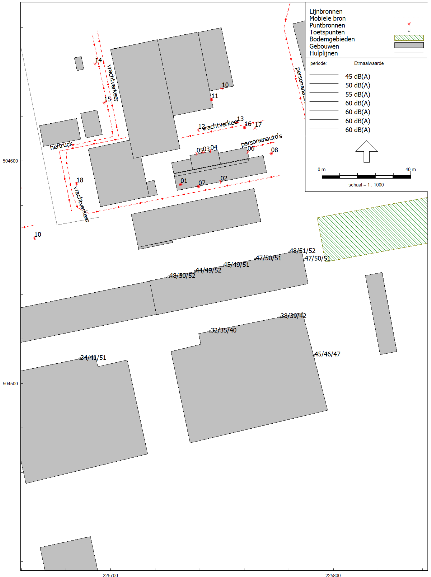
Geluidbelasting verlengde loods met maatregelen etmaalwaarde gecumuleerd zondertoeslag tonaal geluid
