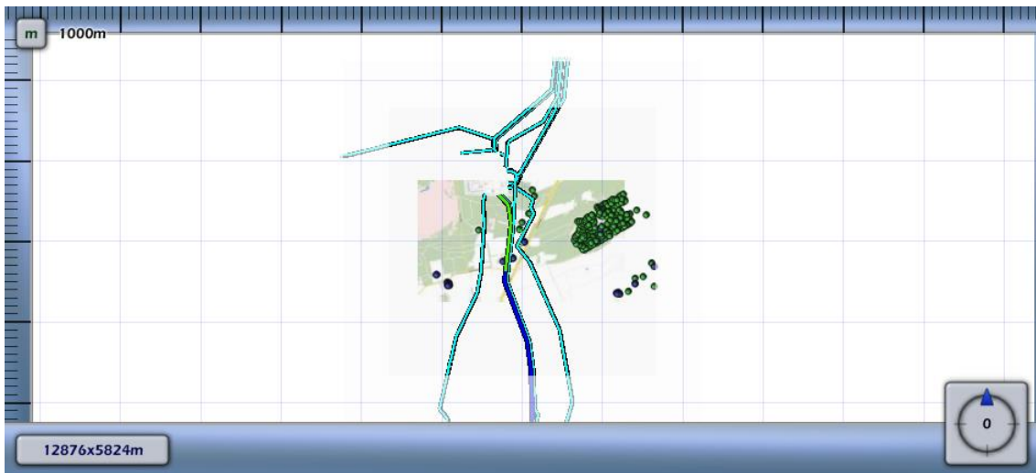
4.7 Figuur 4.7 Groepsrisico screening voor 6165_leiding-A-508-08-deel-1 van N.V. Nederlandse Gasunie
