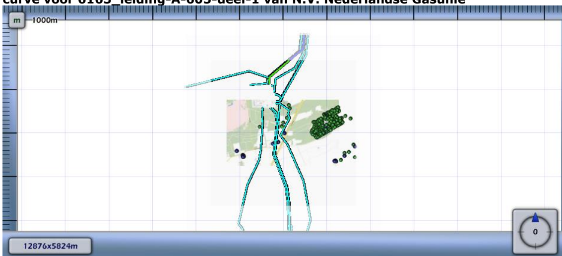
Figuur 4.25 Kilometer leiding behorende bij de maximale overschrijding van de FN-curve voor 6165 leiding-A-605-deel-1 van N.V. Nederlandse Gasunie
