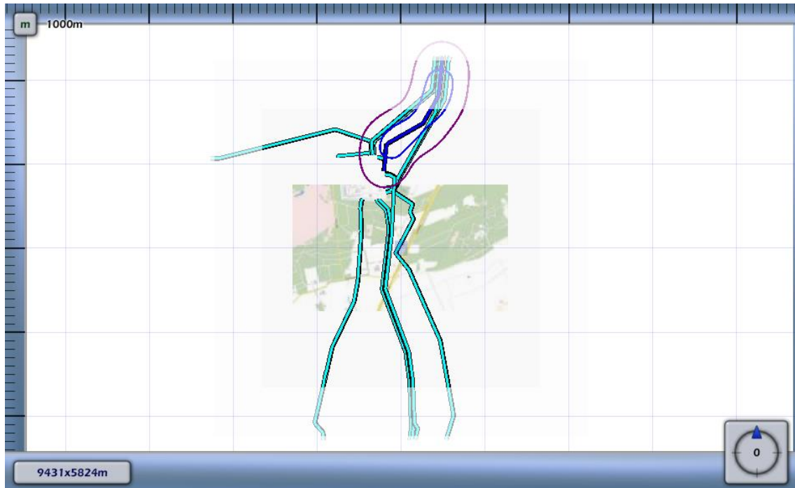
3.5 Figuur 3.5 Plaatsgebonden risico voor 6165_leiding-A-505-deel-1 van N.V. Nederlandse Gasunie
