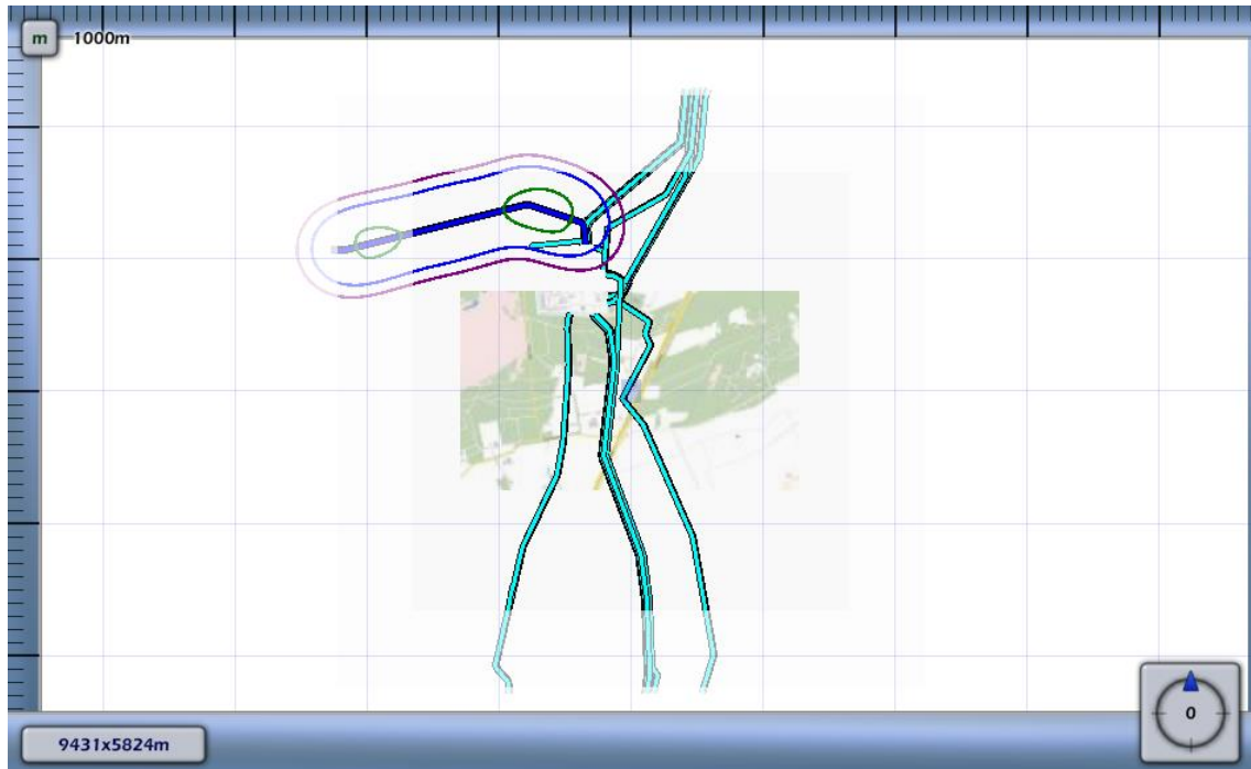
3.13 Figuur 3.13 Plaatsgebonden risico voor 6165_leiding-A-511-deel-1 van N.V. Nederlandse Gasunie
