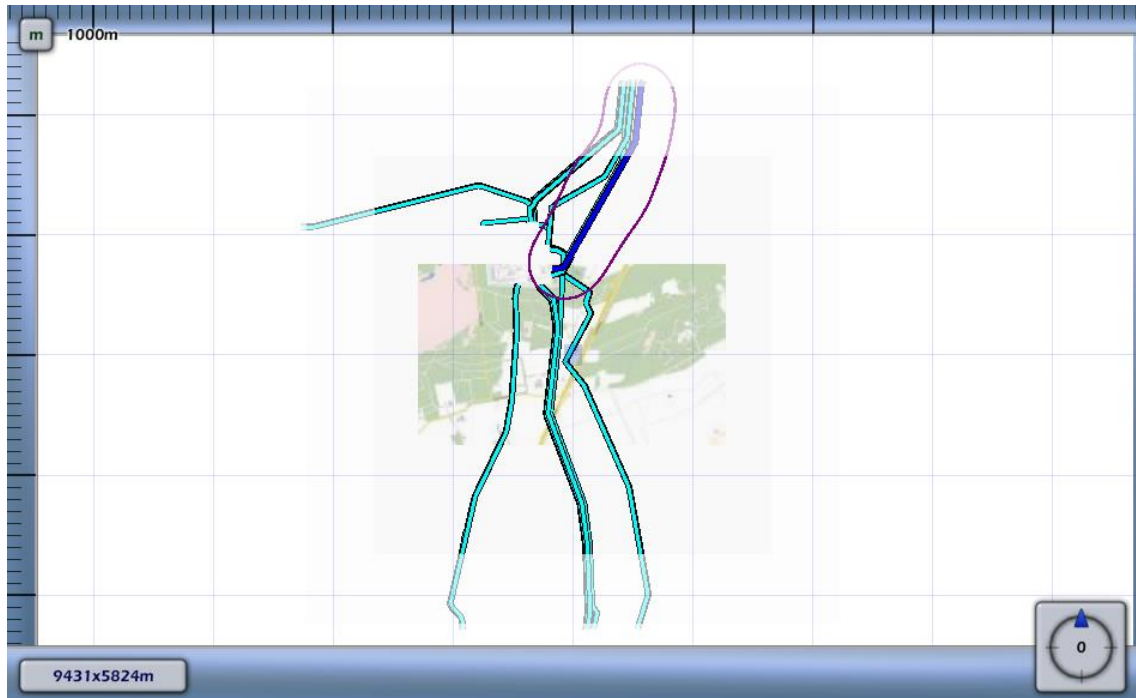
3.19 Figuur 3.19 Plaatsgebonden risico voor 6165_leiding-A-522-deel-1 van N.V. Nederlandse Gasunie
