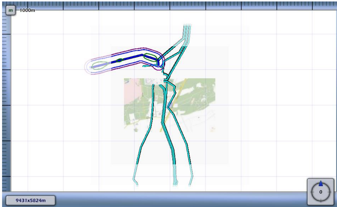
3.25 Figuur 3.25 Plaatsgebonden risico voor 6165_leiding-A-605-deel-1 van N.V. Nederlandse Gasunie
