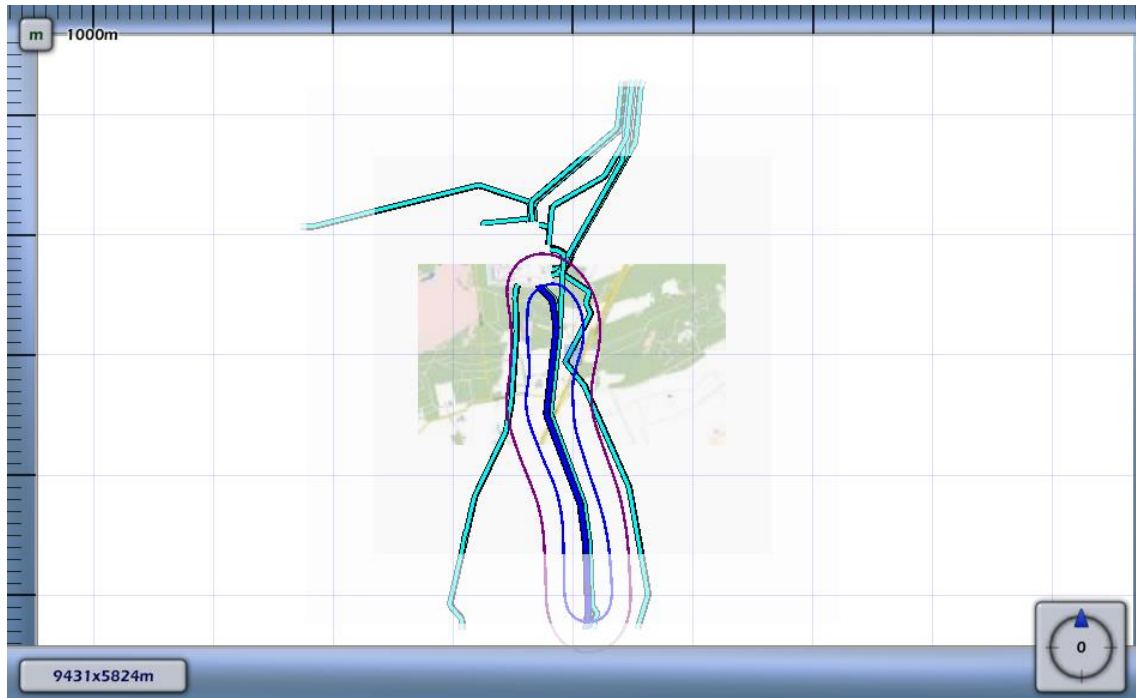
3.7 Figuur 3.7 Plaatsgebonden risico voor 6165_leiding-A-508-08-deel-1 van N.V. Nederlandse Gasunie
