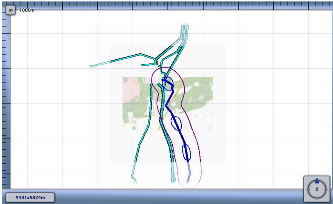
3.21 Figuur 3.21 Plaatsgebonden risico voor 6165_leiding-A-529-deel-1 van N.V. Nederlandse Gasunie
