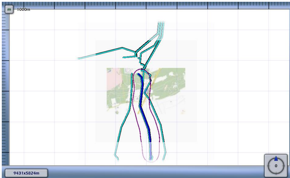
3.23 Figuur 3.23 Plaatsgebonden risico voor 6165_leiding-A-588-deel-1 van N.V. Nederlandse Gasunie
