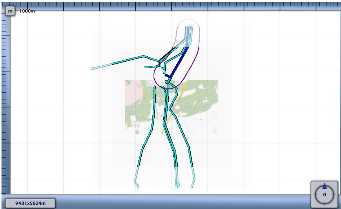
3.29 Figuur 3.29 Plaatsgebonden risico voor 6165_leiding-A-661-deel-1 van N.V. Nederlandse Gasunie
