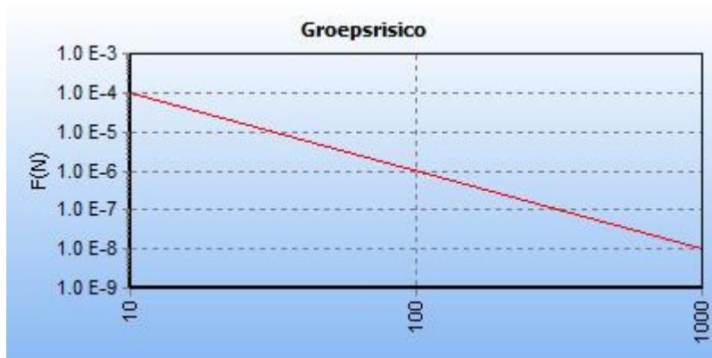
5.17 Figuur 5.17 FN curve voor 6165_leiding-A-519-05-deel-1 van N.V. Nederlandse Gasunie voor de kilometer tussen stationing 0.00 en stationing 180.00
