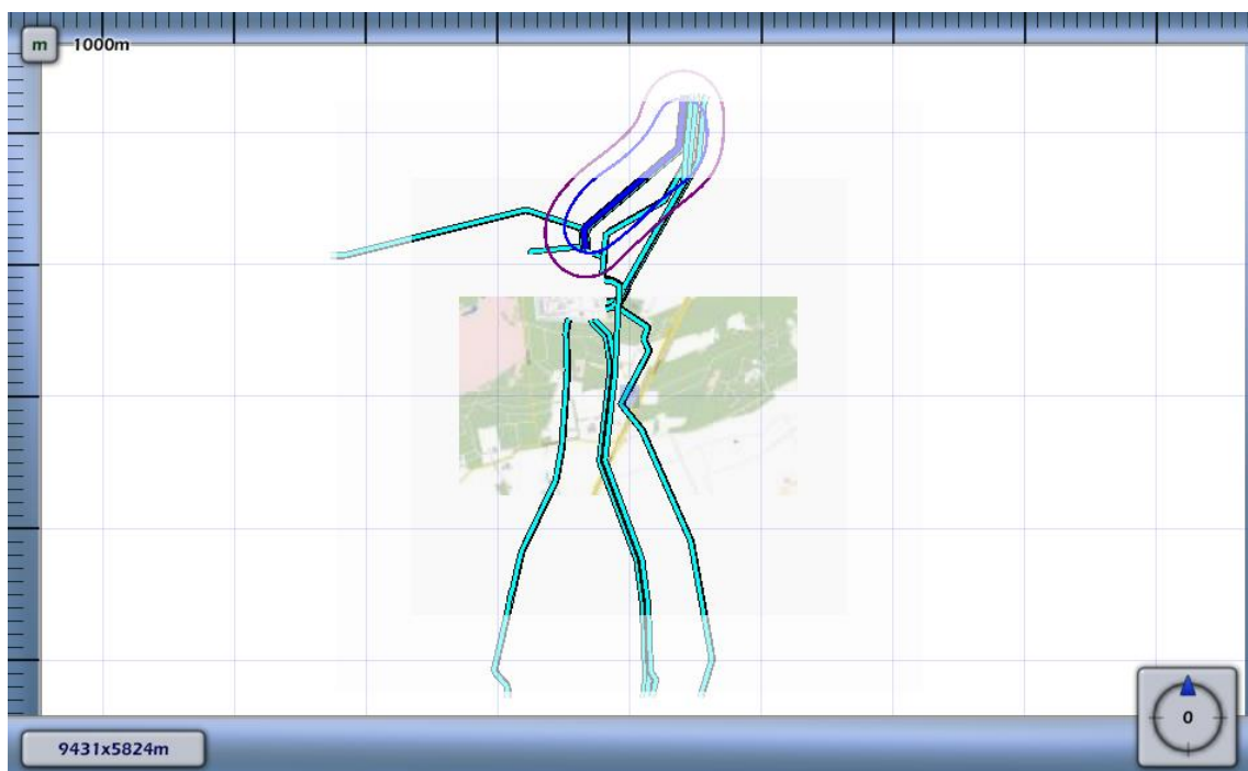
3.1 Figuur 3.1 Plaatsgebonden risico voor 6165_leiding-A-501-deel-1 van N.V. Nederlandse Gasunie
