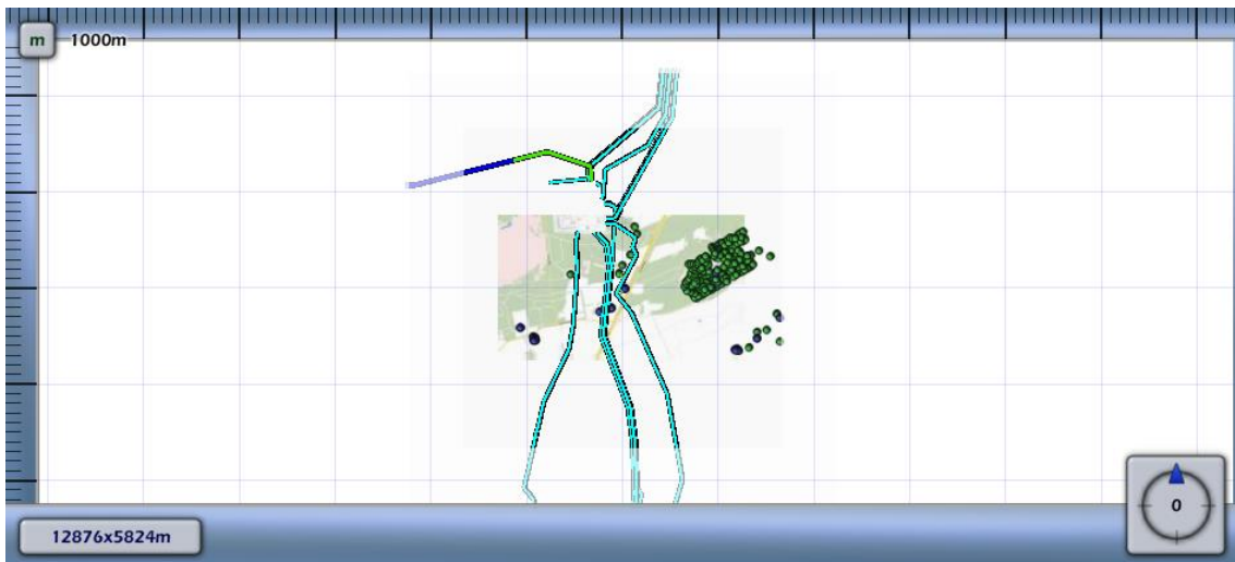
4.25 Figuur 4.25 Groepsrisico screening voor 6165_leiding-A-605-deel-1 van N.V. Nederlandse Gasunie
