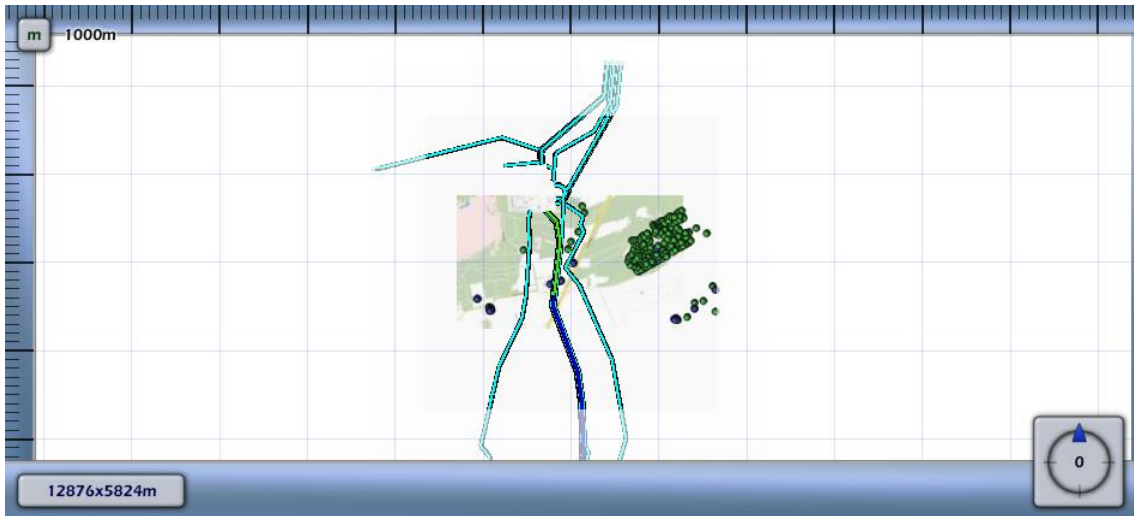
4.10 Figuur 4.10 Groepsrisico screening voor 6165_leiding-A-509-09-deel-1 van N.V. Nederlandse Gasunie
