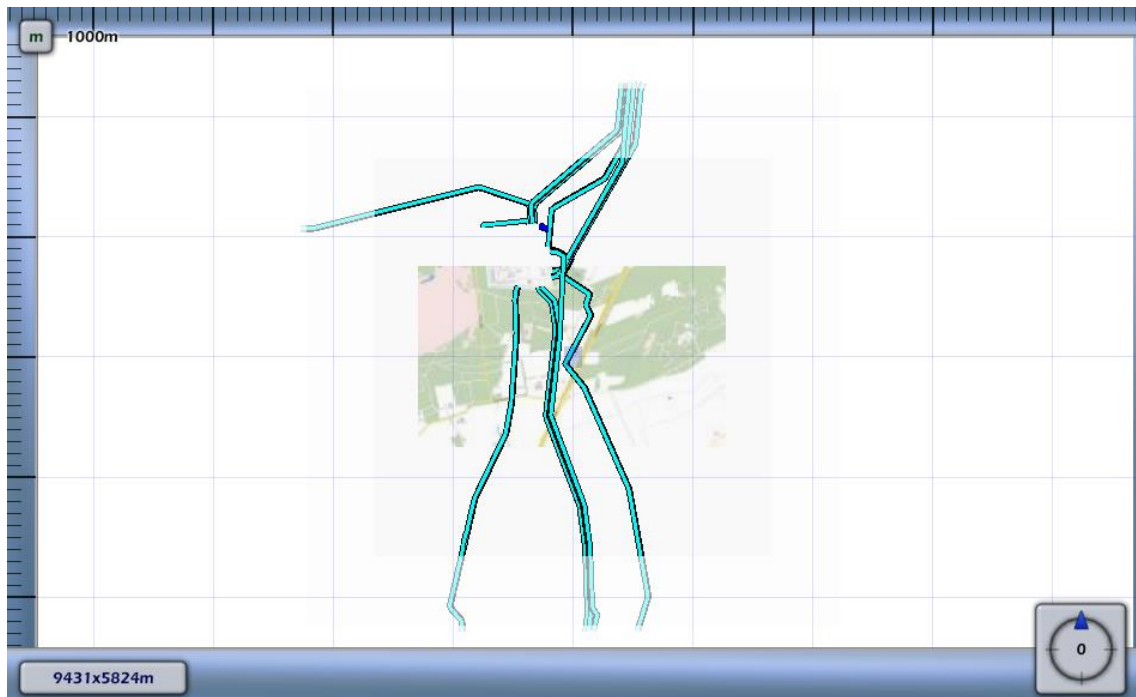
3.3 Figuur 3.3 Plaatsgebonden risico voor 6165_leiding-A-503-07-deel-1 van N.V. Nederlandse Gasunie
