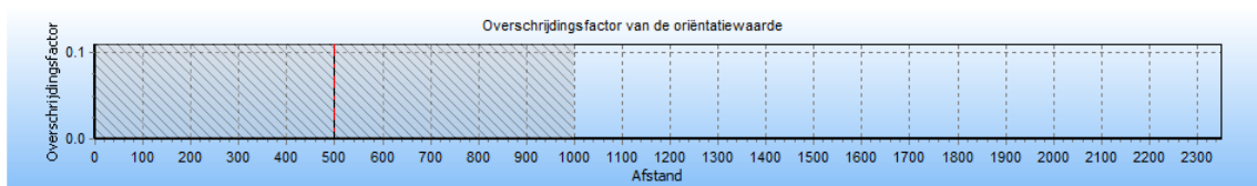
4.22 Figuur 4.22 Groepsrisico screening voor 6165_leiding-A-549-deel-1 van N.V. Nederlandse Gasunie
