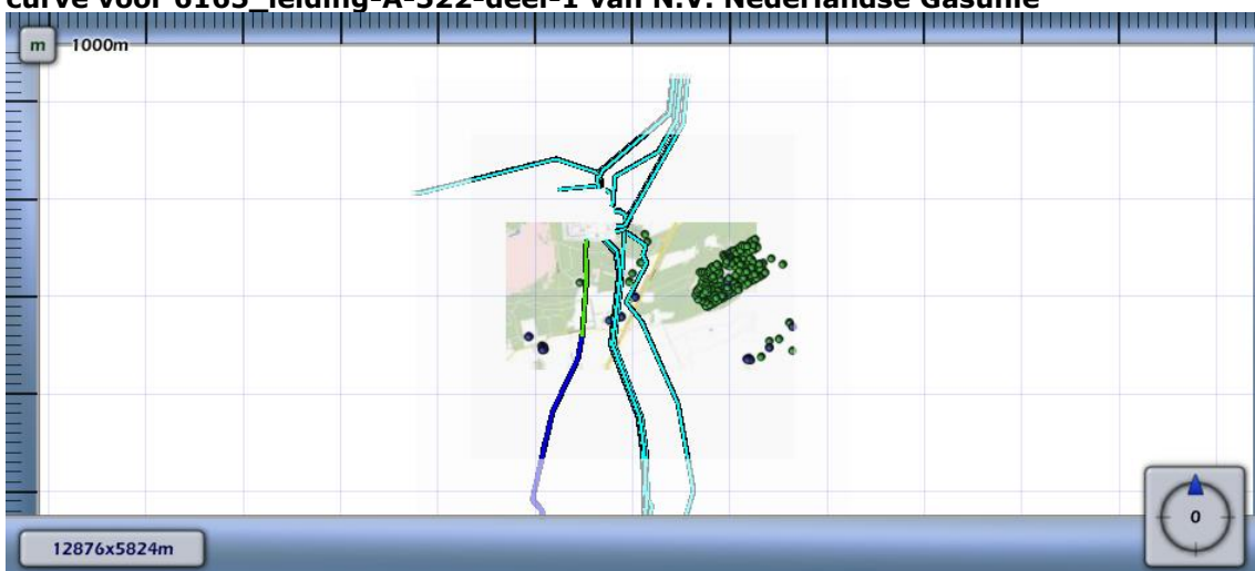
Figuur 4.19 Kilometer leiding behorende bij de maximale overschrijding van de FN-curve voor 6165_leiding-A-522-deel-1 van N.V. Nederlandse Gasunie
