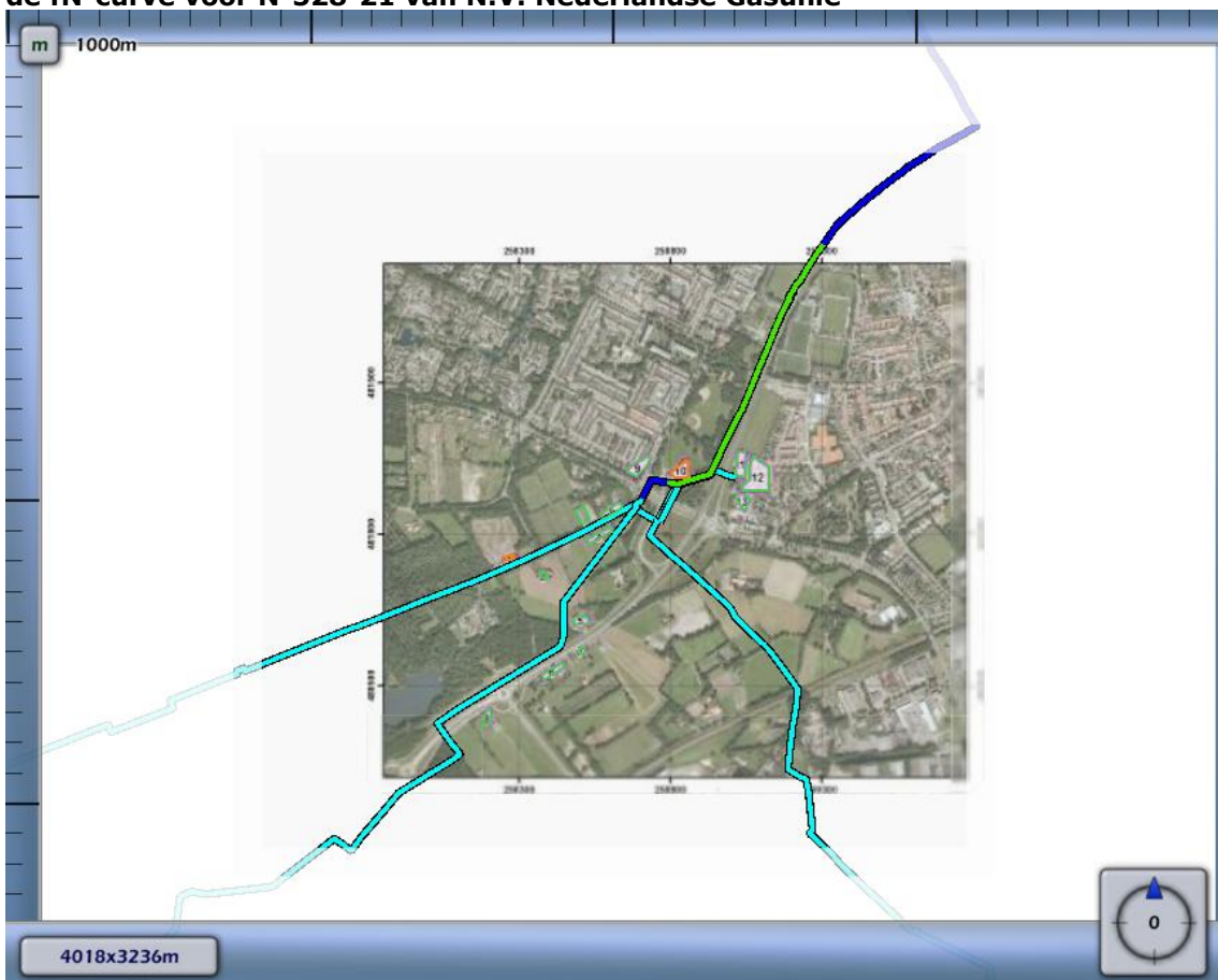
Figuur 4.2 Kilometer leiding (groen) behorende bij de maximale overschrijding van de fN-curve voor N-528-21 van N.V. Nederlandse Gasunie
