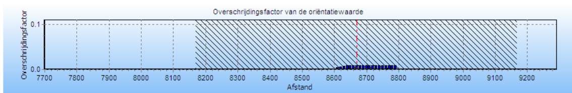
Figuur 4.2 Groepsrisico screening voor N-528-21 van N.V. Nederlandse Gasunie
