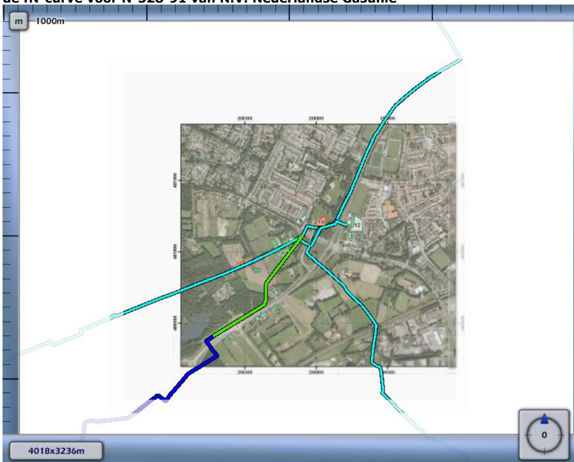
Figuur 4.1 Kilometer leiding (groen) behorende bij de maximale overschrijding van de fN-curve voor N-528-91 van N.V. Nederlandse Gasunie
