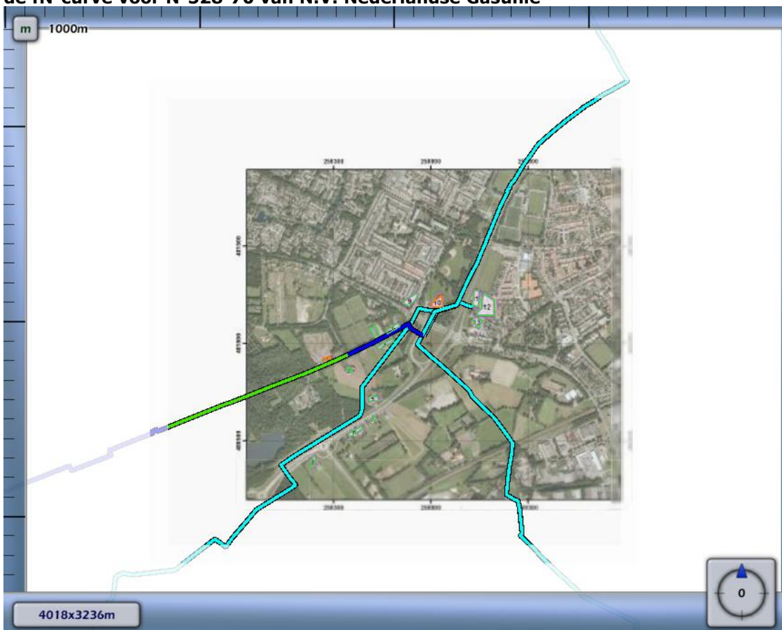
Figuur 4.4 Kilometer leiding (groen) behorende bij de maximale overschrijding van de fN-curve voor N-528-70 van N.V. Nederlandse Gasunie
