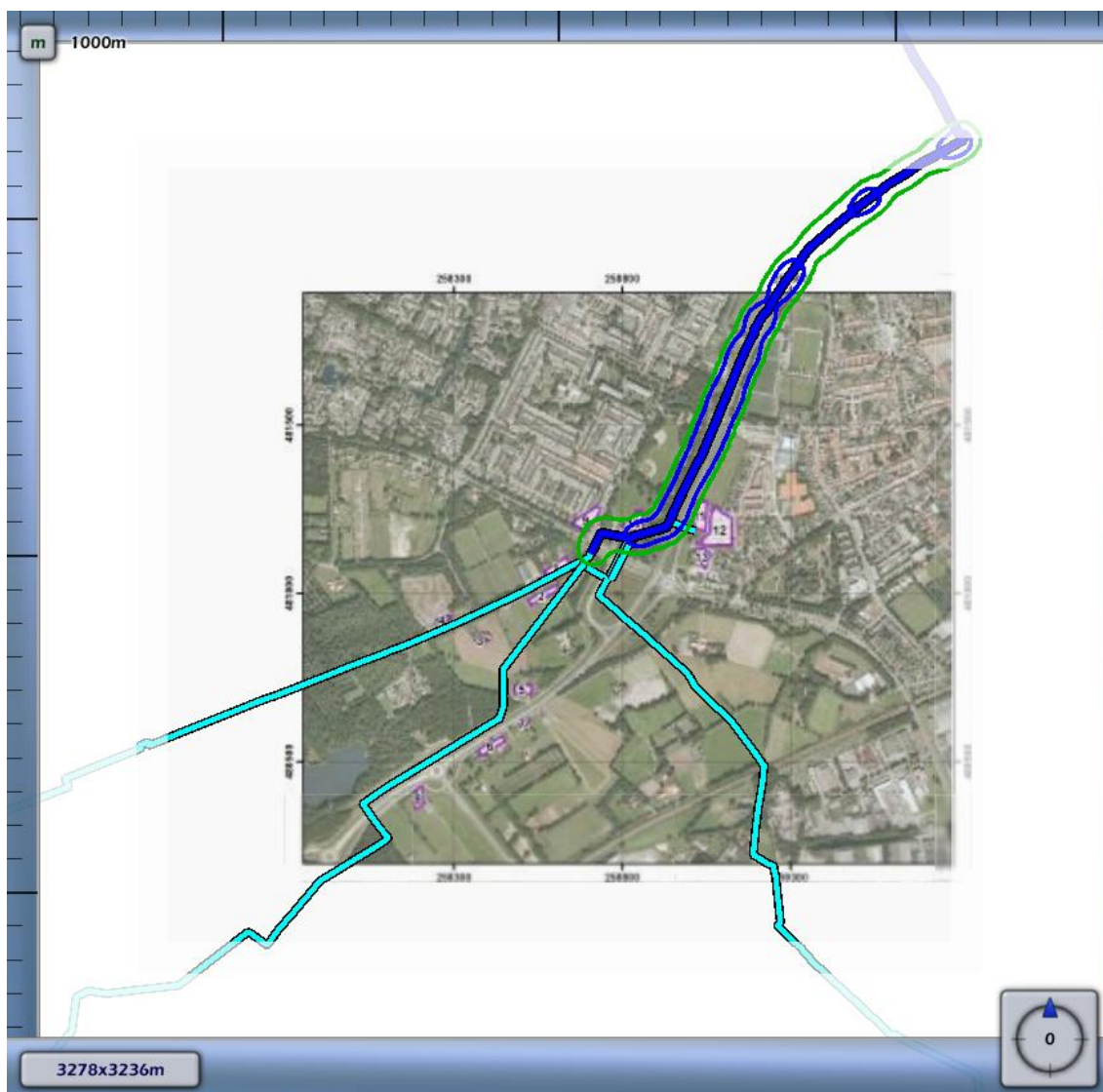
Figuur 3.2 Plaatsgebonden risico voor N-528-21 van N.V. Nederlandse Gasunie
