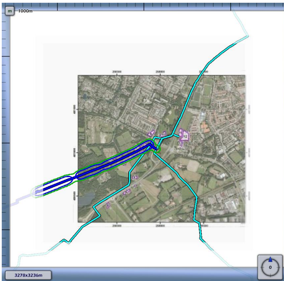
Figuur 3.4 Plaatsgebonden risico voor N-528-70 van N.V. Nederlandse Gasunie
