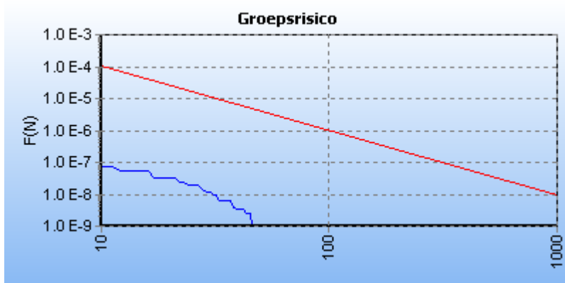
Figuur 5.1 FN curve voor N-528-91 van N.V. Nederlandse Gasunie voor de kilometer tussen stationing 690.00 en stationing 1690.00
