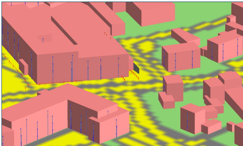
Figuur 7 Impressie rekenmodel met scherm
