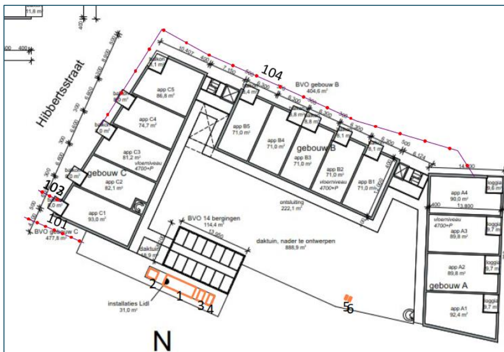
Figuur 3 Situering installaties en ligging rijroutes
