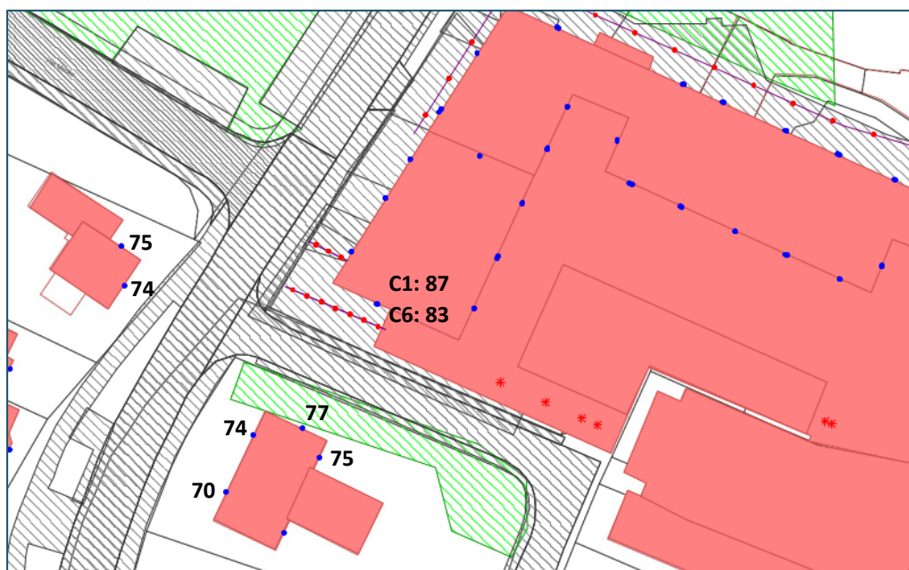
Figuur 5 Optredende maximale geluidsniveaus in dagperiode vanwege vrachtwagens zonder scherm
