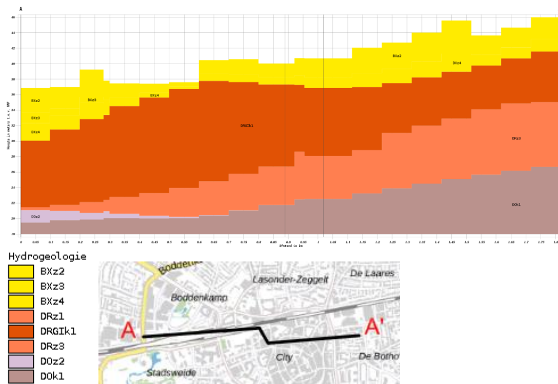
Afbeelding 2.3: Geohydrologische schematisatie van de ondergrond op de locatie (bron: 5).
