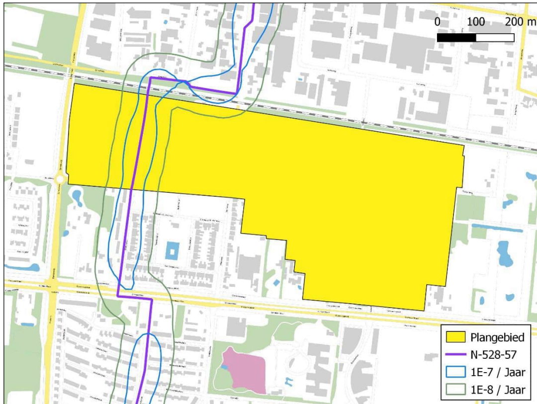
Figuur 3. Plaatsgebonden risicocontouren aardgasleiding N-528-57
