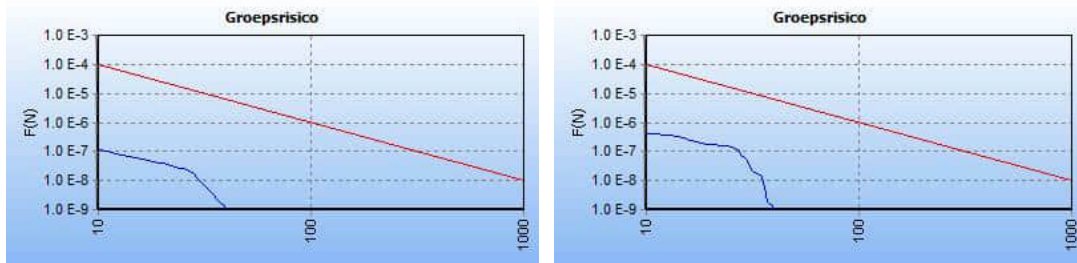
Figuur 4. Groepsrisico N-528-50, huidige (links) en toekomstige situatie (rechts)
