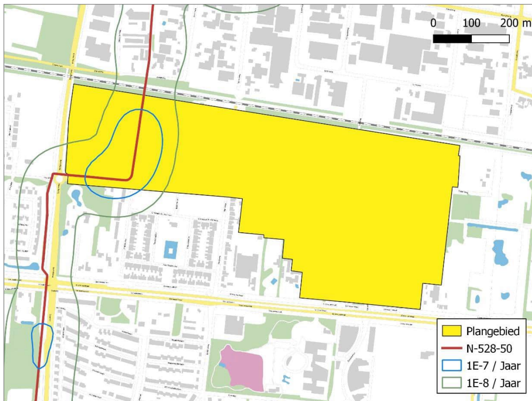
Figuur 2. Plaatsgebonden risicocontouren aardgasleiding N-528-50
