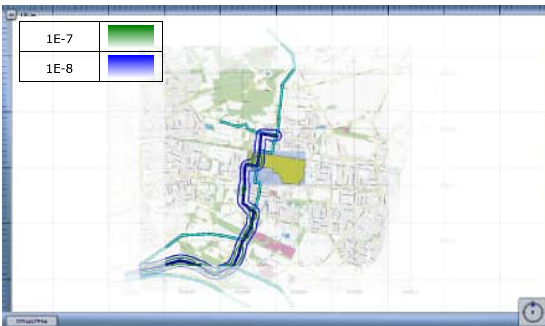
3.2 Figuur 3.2 Plaatsgebonden risico voor 8934_leiding-N-528-57-deel-1 van N.V. Nederlandse Gasunie
