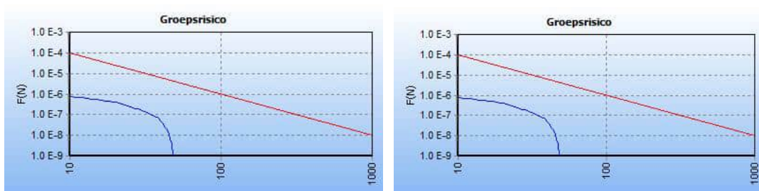
Figuur 5. Groepsrisico N-528-57, huidige (links) en toekomstige situatie (rechts)
