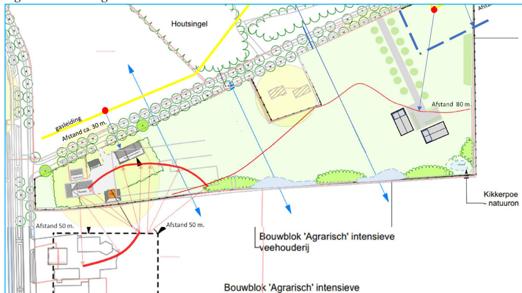
Figuur 1: inrichtingsschets
