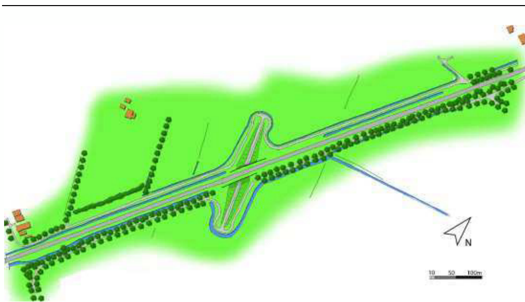
Figuur 4.21_Nieuwe situatie in bouwsteen 10
