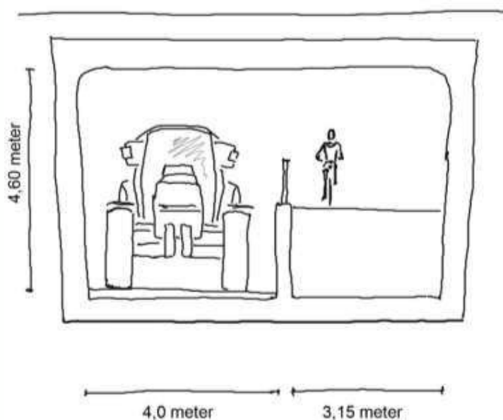
Figuur 4.22 Principeprofiel van de tunnel
