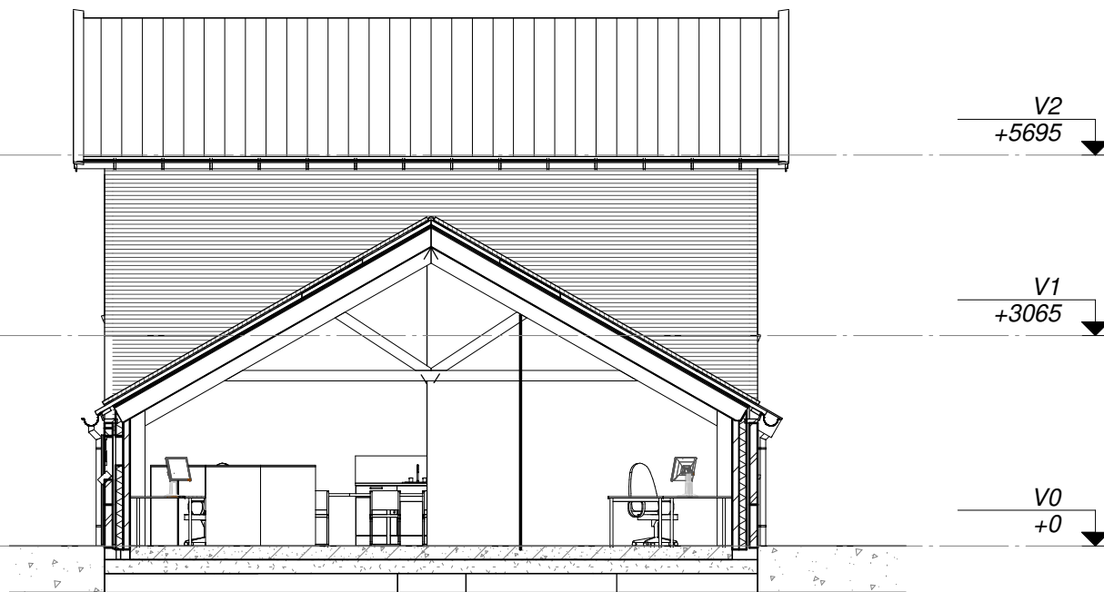
doorsnede B-B
