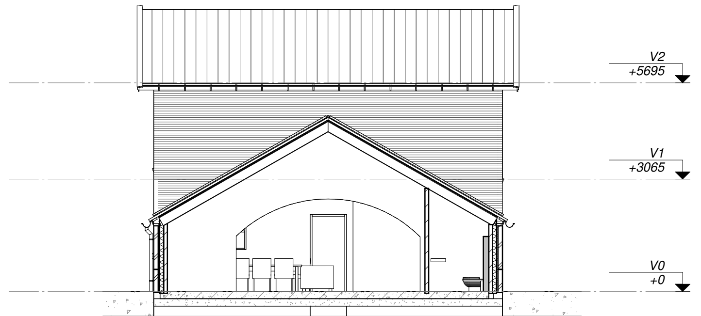
doorsnede C-C
