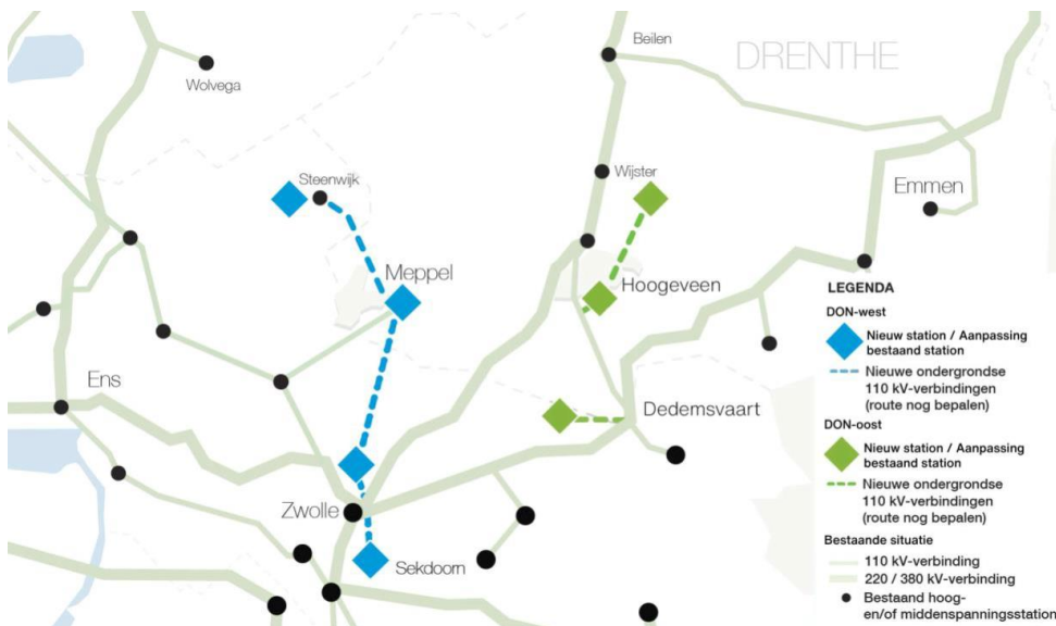
Figuur 1.2 | Overzicht werkzaamheden uitbreiding elektriciteitsnet Noordwest Overijssel en Zuidwest Drenthe
