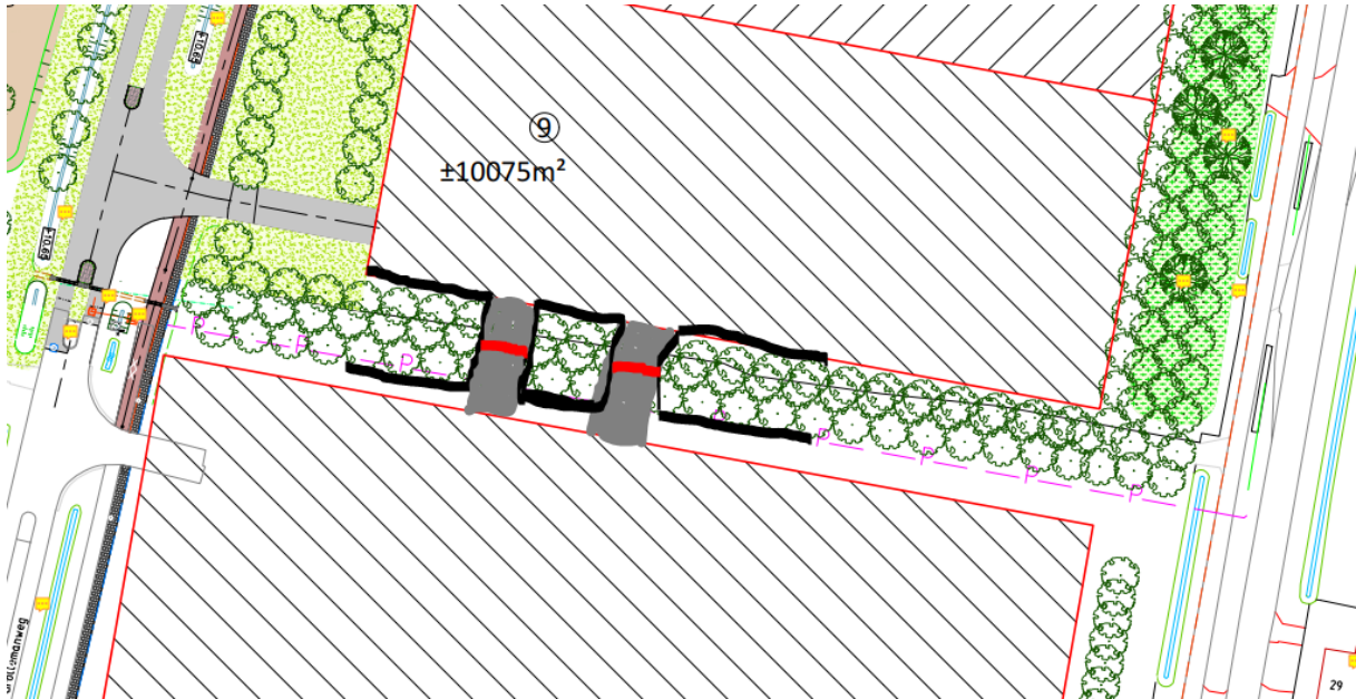
Schets van het plangebied, met daarin de faunapassages (rode lijn) en geleiding (zwarte lijn) ingetekend. De geleiding is ten minste 30 meter lang
