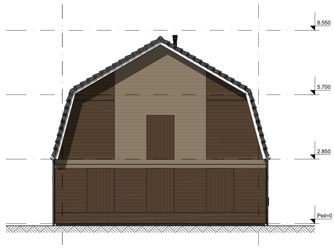
Linker gevel
