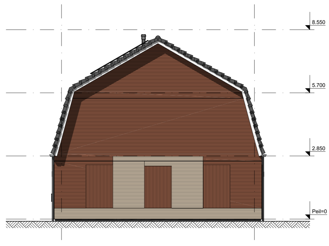
Rechtergevel
