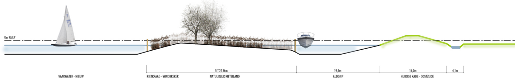
DWARSDOORSNEDE TER HOOGTE VAN DE OOSTELIJKE OEVER
