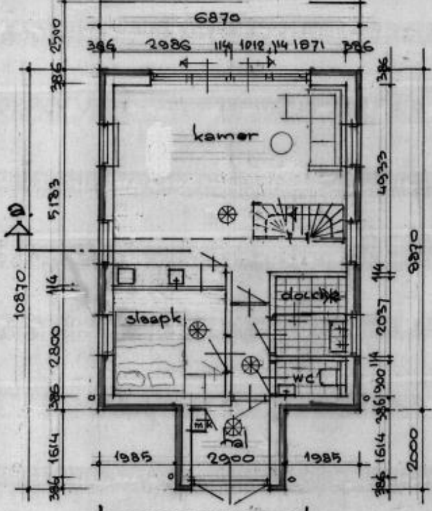
begane grond. verdieping. PLATTEGRONDEN MET Aangepaste maatvoering
