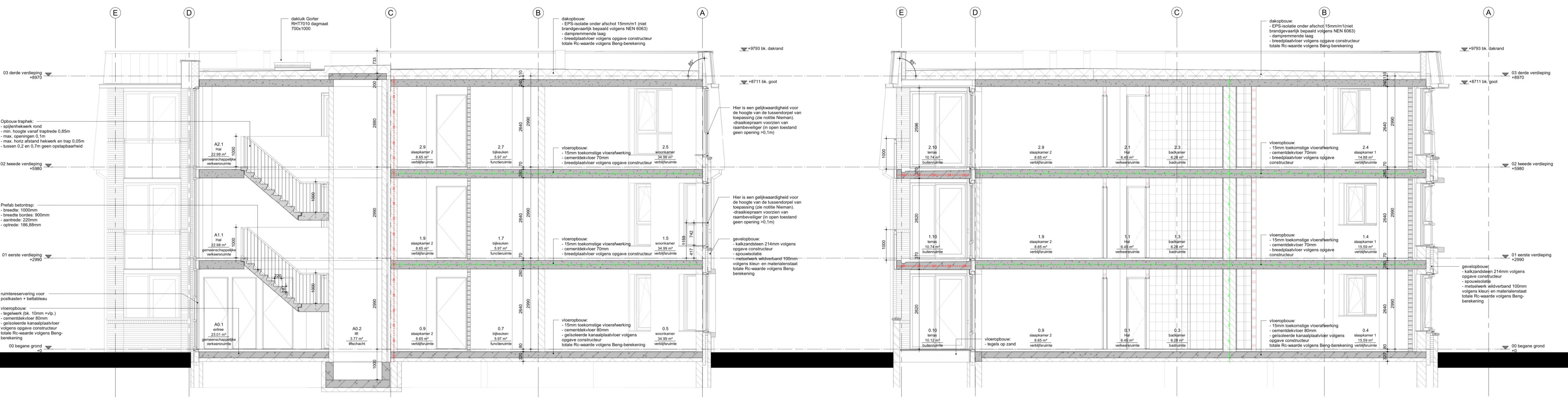
Doorsnede A-A 1 : 50
