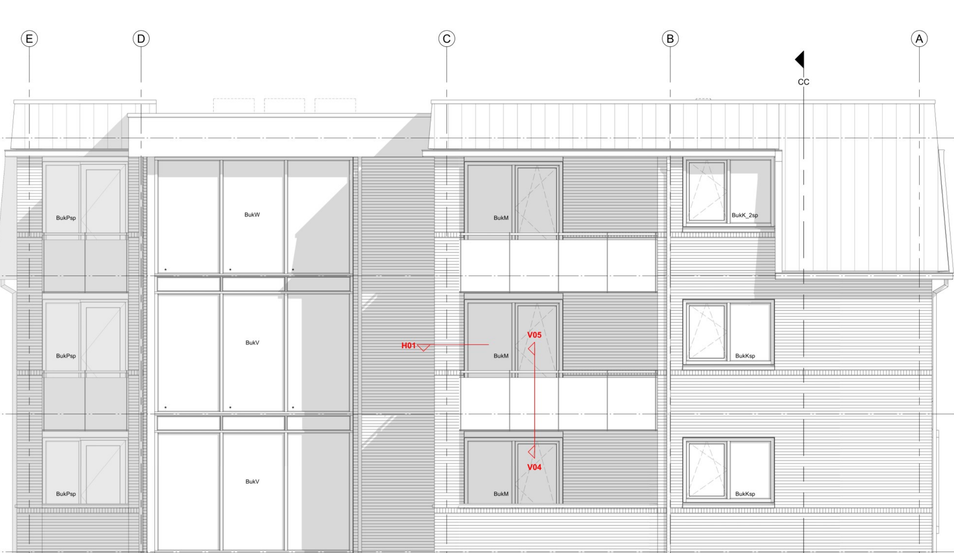
Zuidgevel
