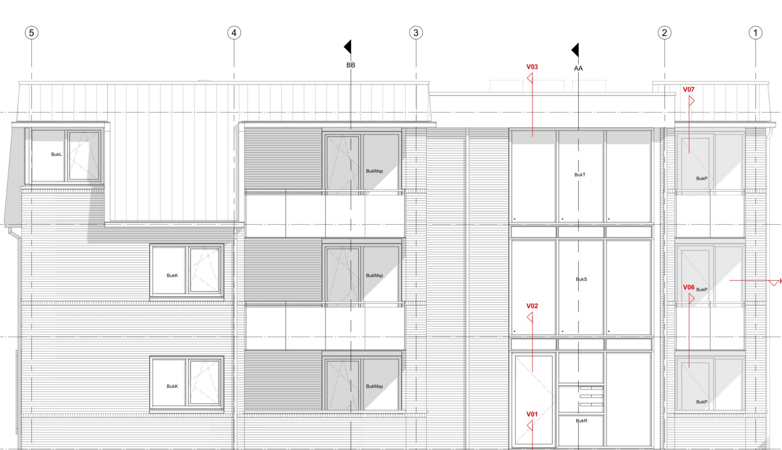
Westgevel
