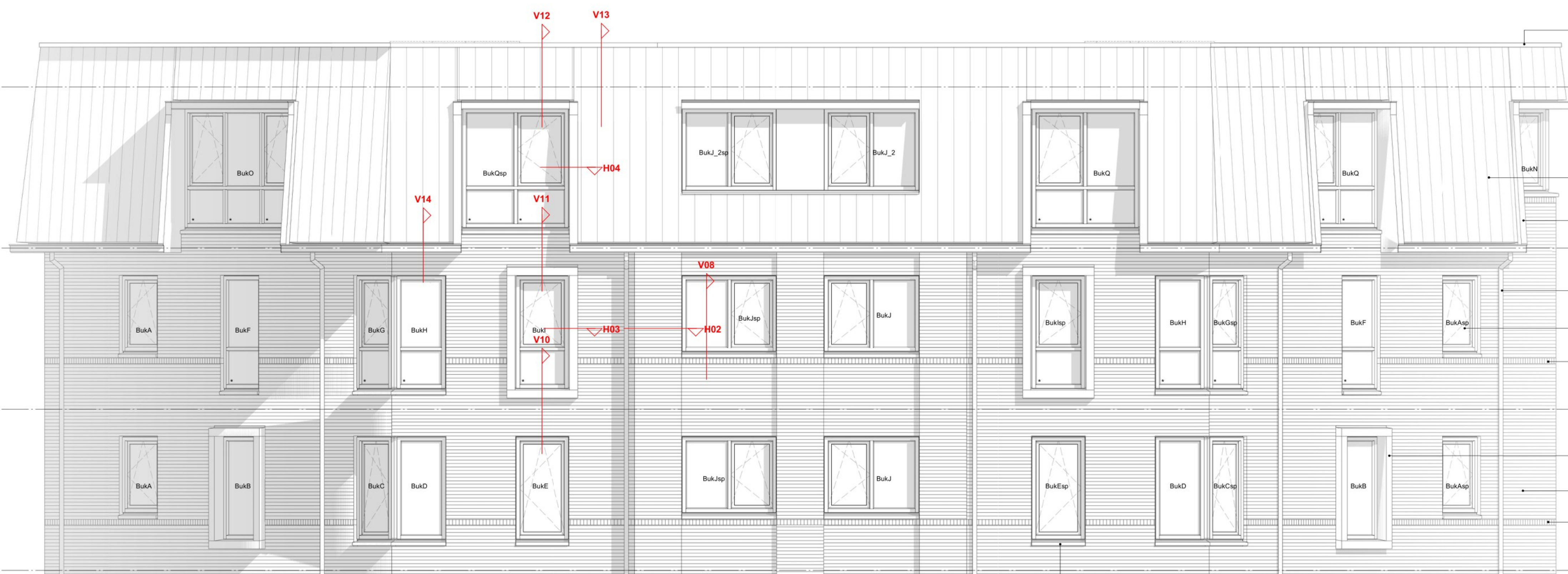
Noordoostgevel
