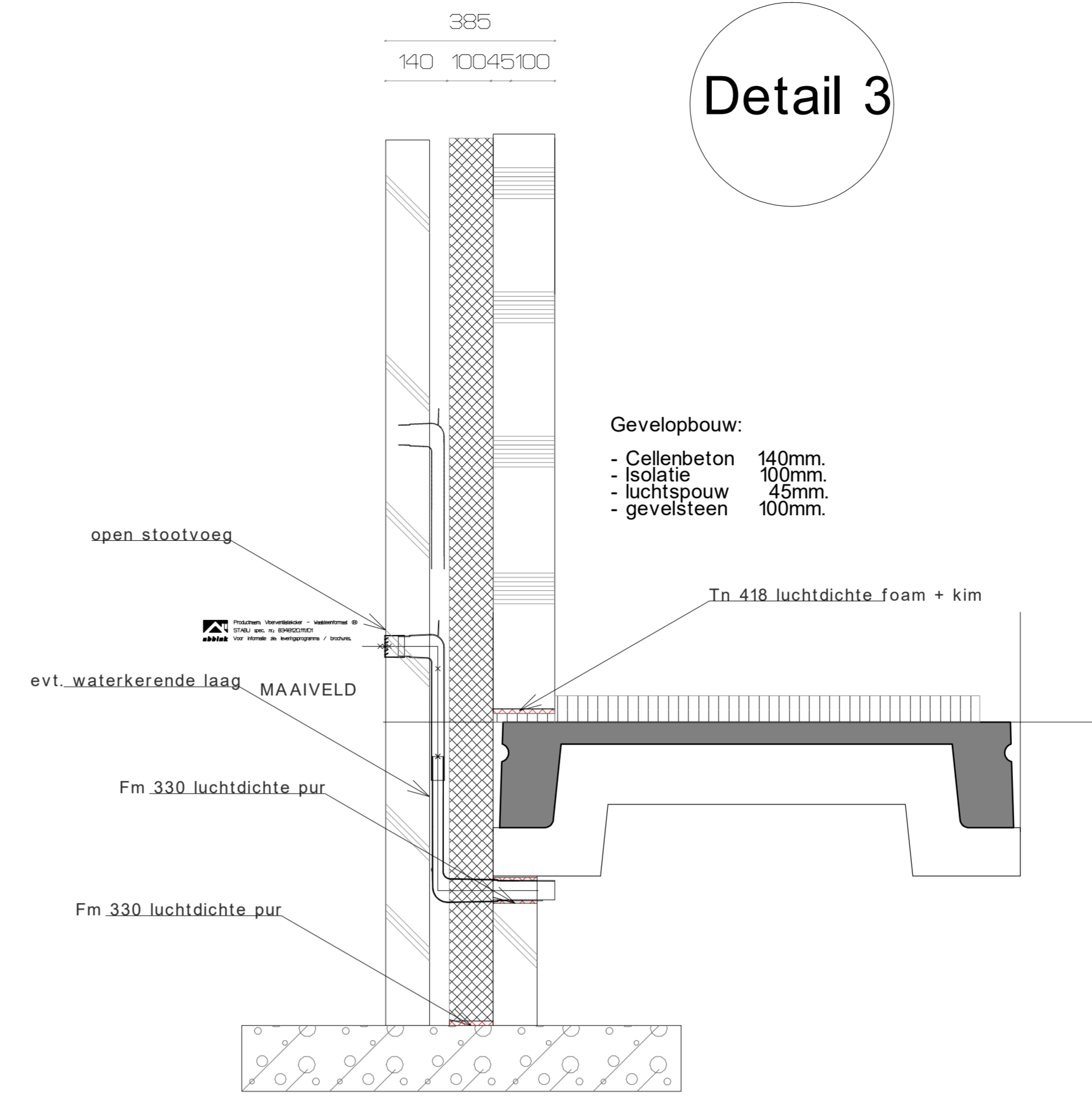
Luchtdichte detailering peil
