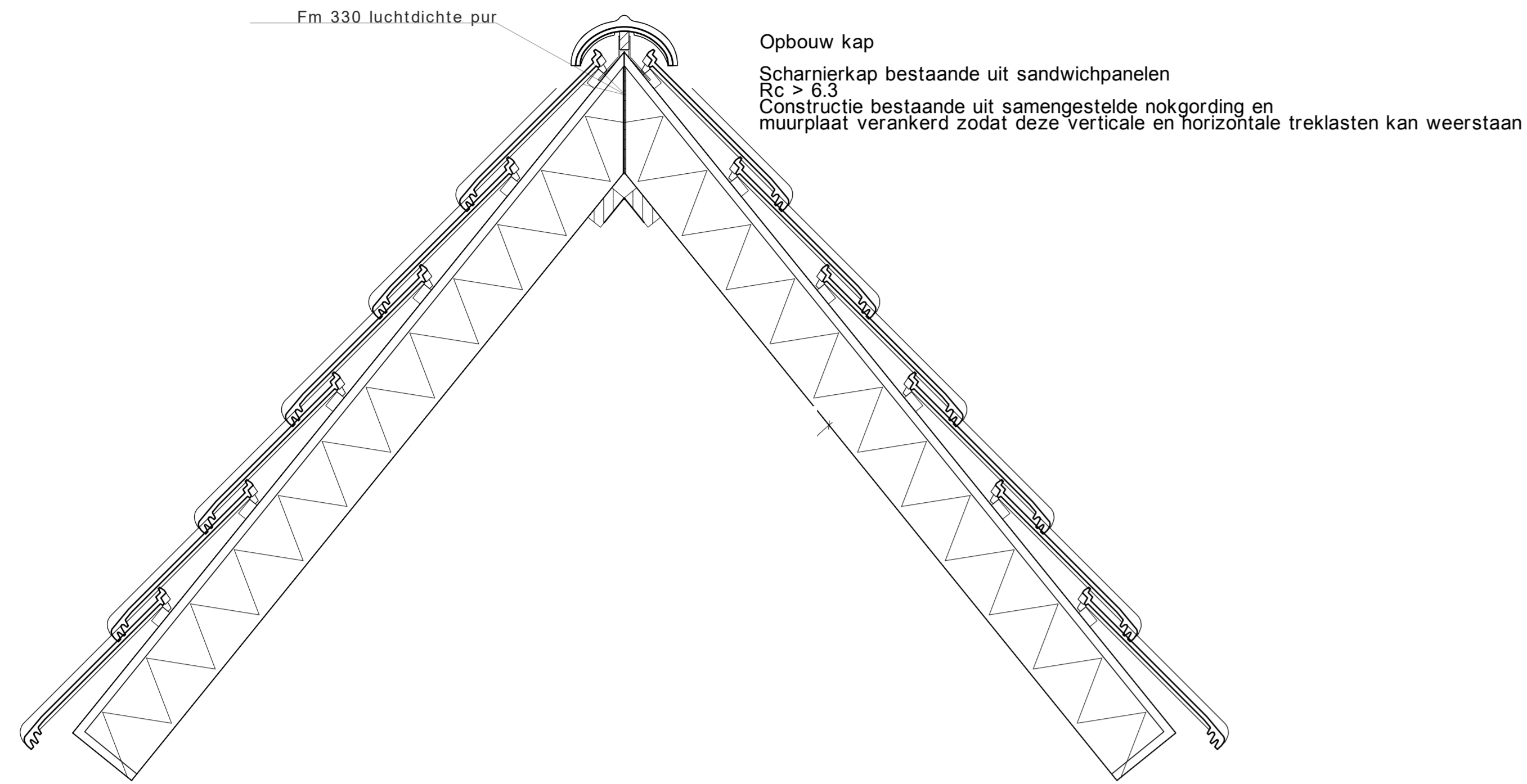
Luchtdichte detailering kap
