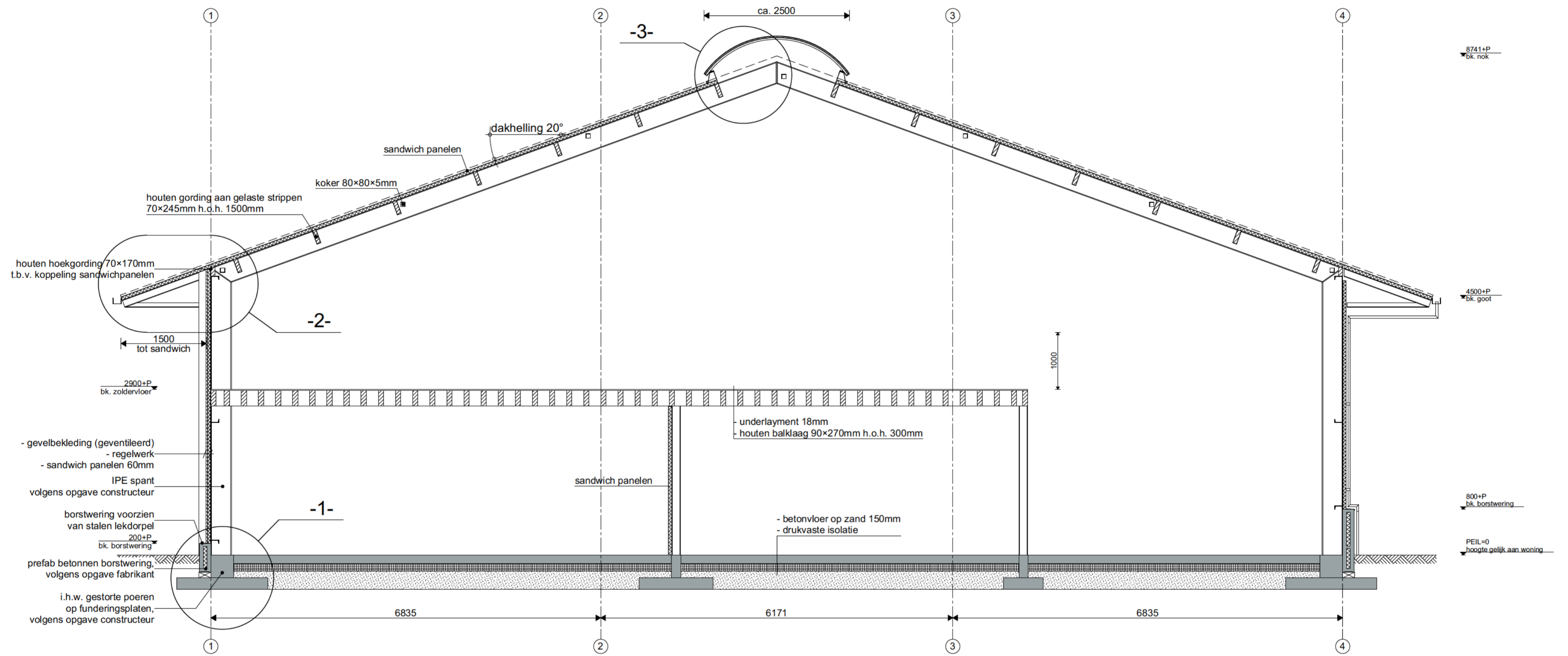
Doorsnede B-B
