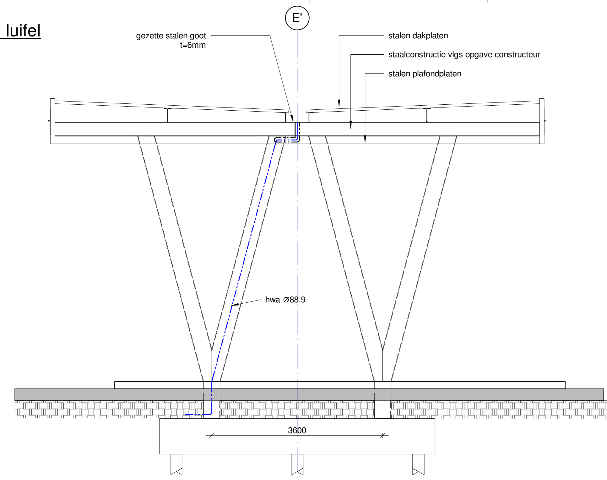
Dwarsdoorsnede luifel
