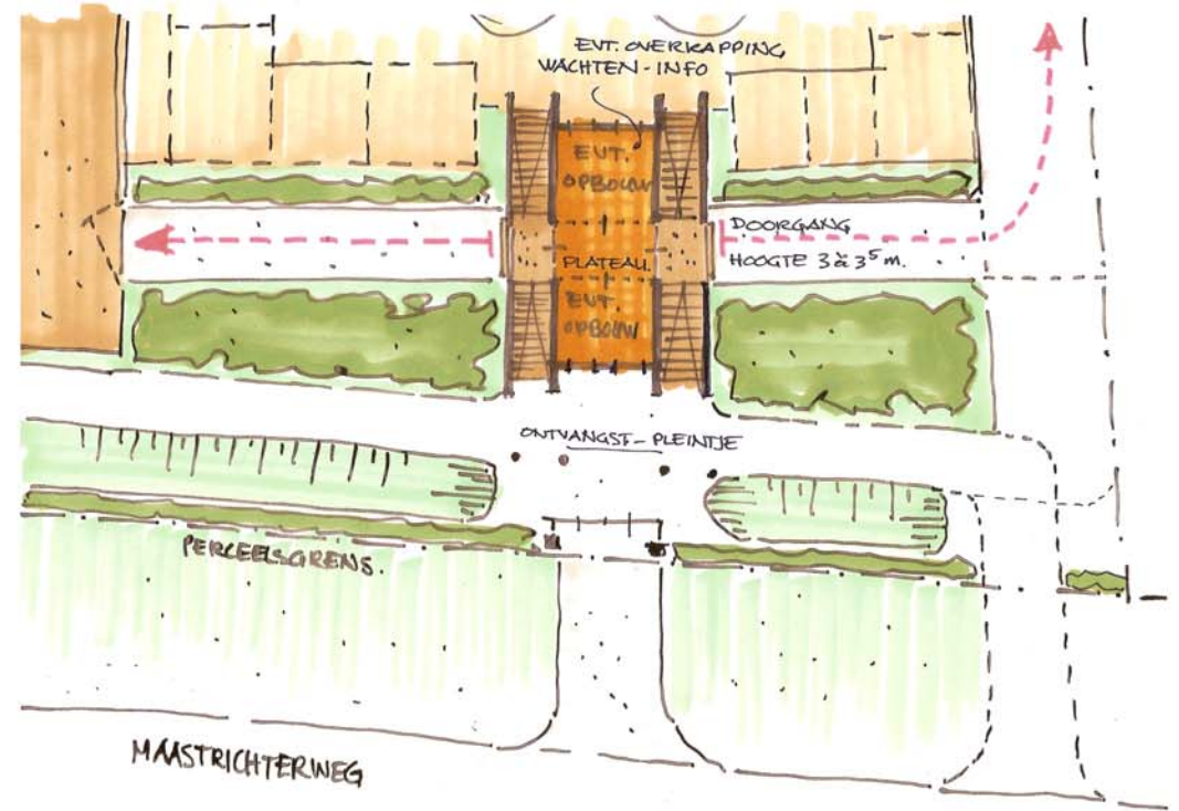
PLATTEGROND 1e VERDIEPING
