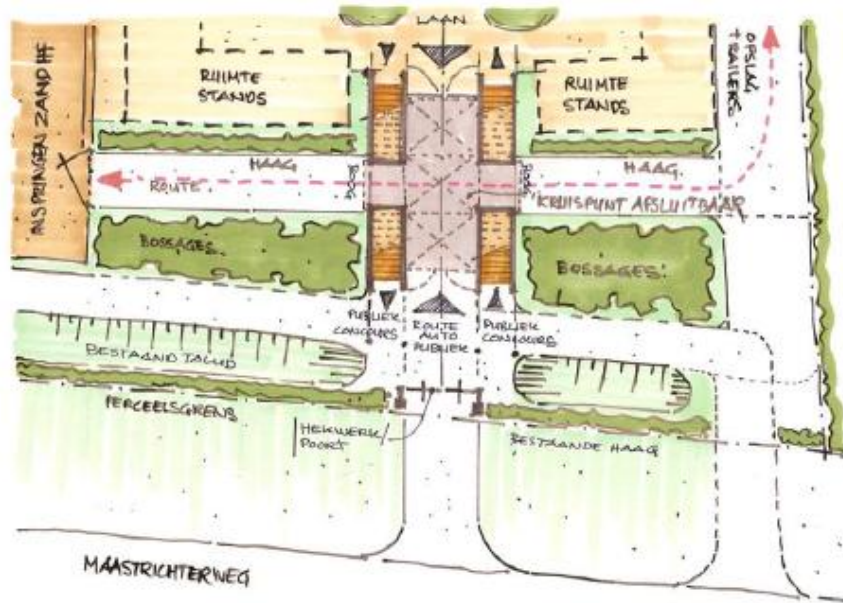
PLATTEGROND BEGANE GROND
