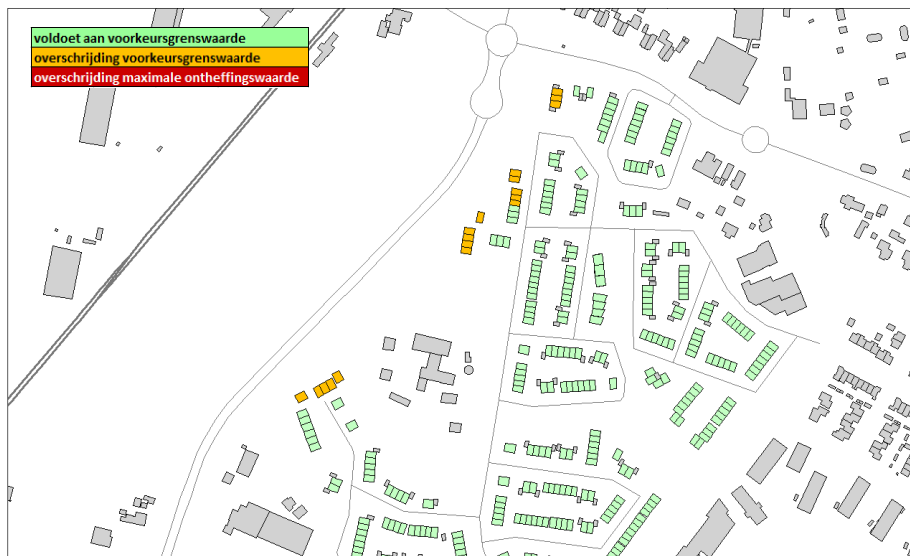
Figuur 5.2: Geluidsbelasting t.g.v. verlengde Henslare (incl. correctie art. 110g Wgh.)
