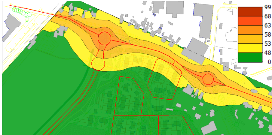
Figuur 5.3: Geluidscontouren vrije veld t.g.v. Stationsstraat (incl. correctie art. 110g Wgh.)
