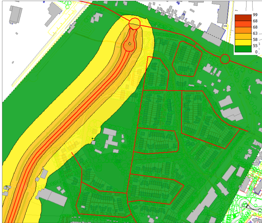
Figuur 5.1: Geluidscontouren vrije veld t.g.v. verlengde Henslare (incl. correctie art. 110g Wgh.)
